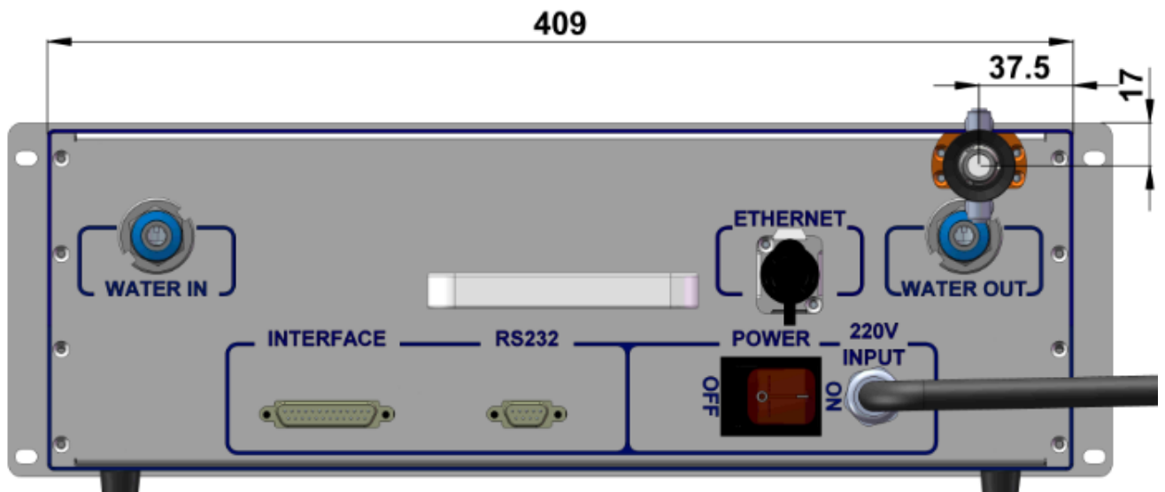
图 2 (b)后视图(单位: mm)
