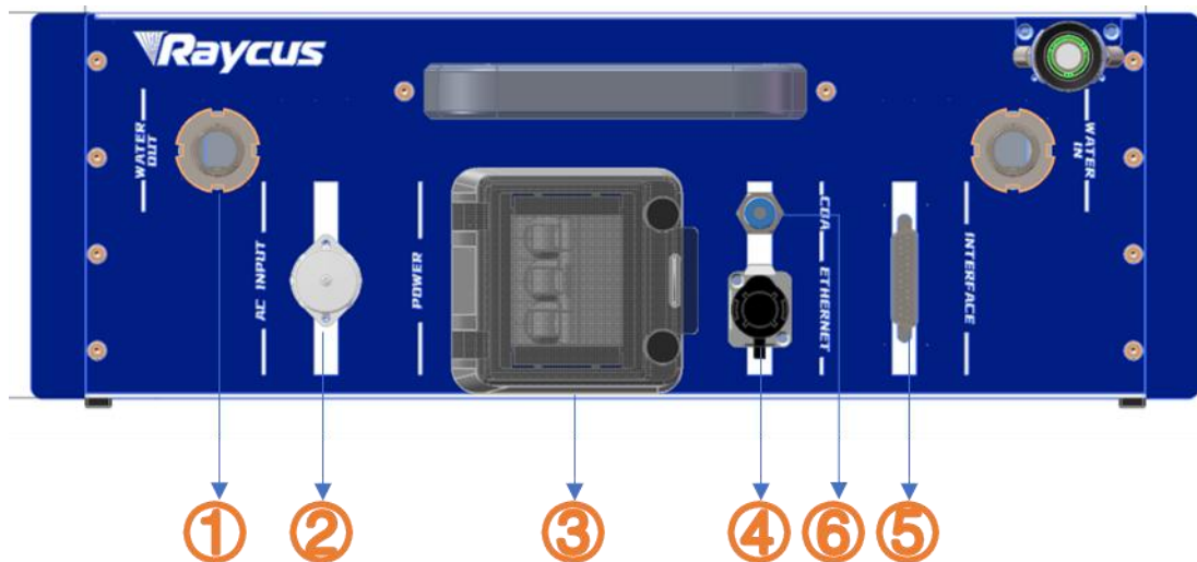
图 5 RFL-C3000S 激光器后面板
