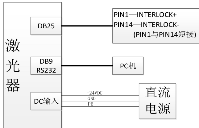
图 10 RS232 模式接线
