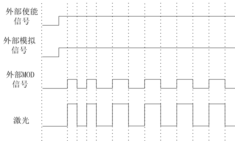
图 9 脉冲工作模式时序
