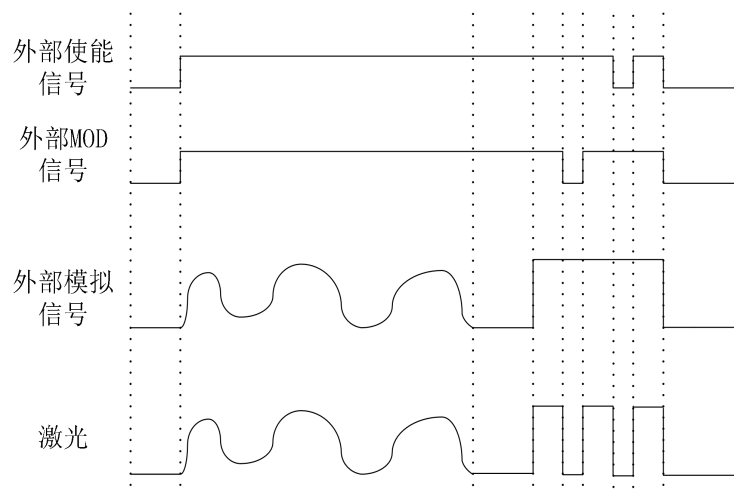
图 8 连续工作模式时序
