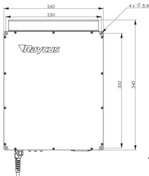
图 2 激光器外形及安装尺寸
