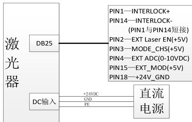
图 7 连续工作模式接线
