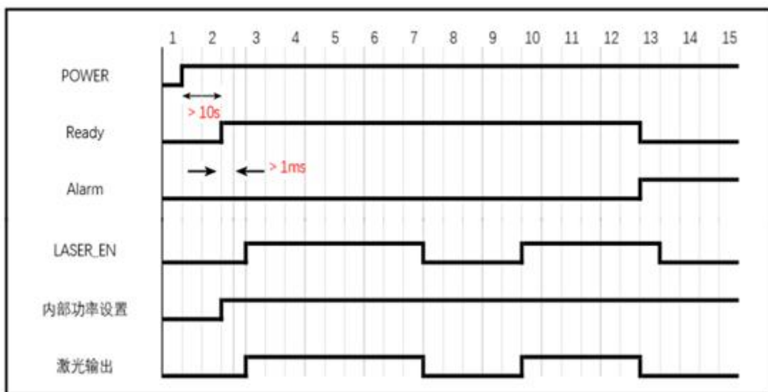
图 22 内控控制方式连续模式时序图
