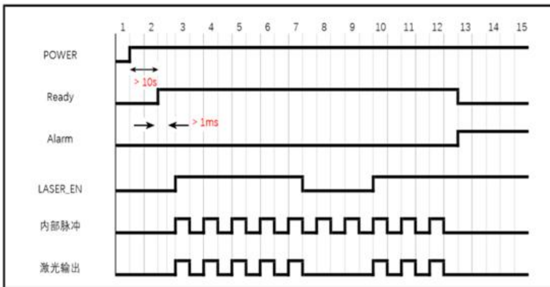
图 23 内控控制方式调制模式时序图
