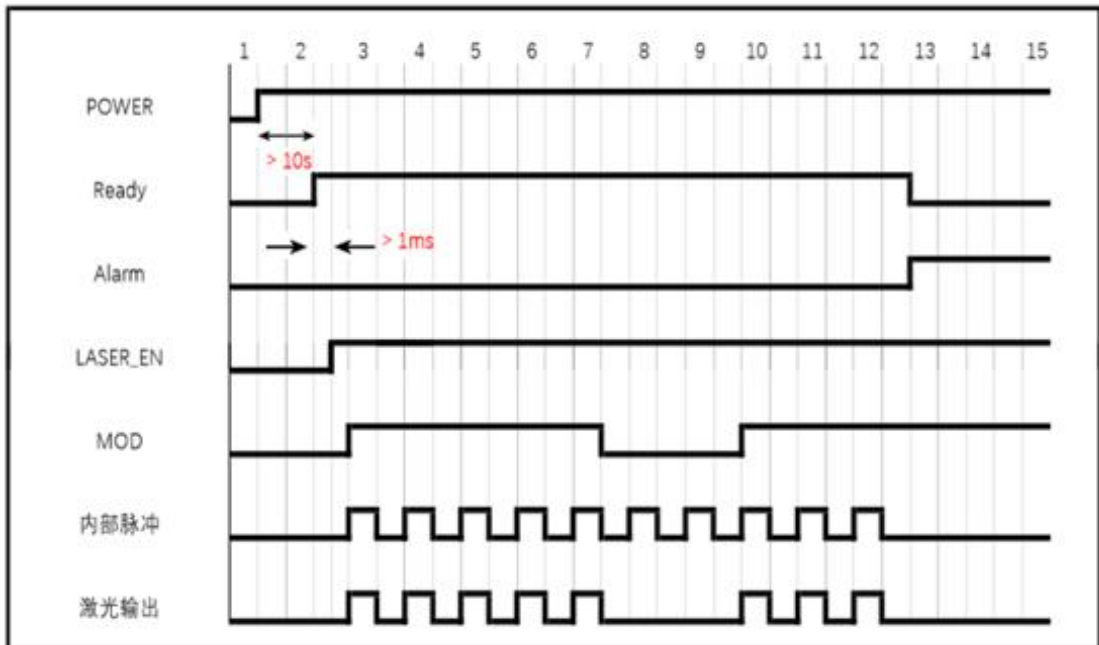
图 18 外控 RS232 控制方式调制模式时序图
