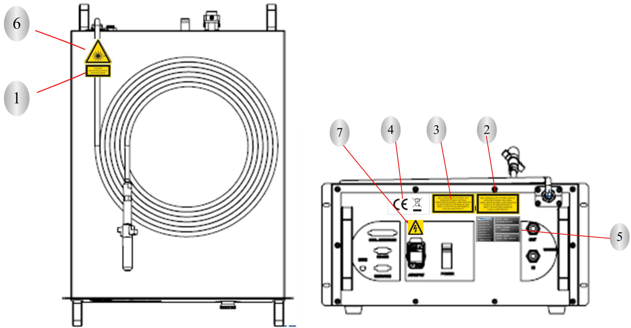
图 1 顶视图及后视图
