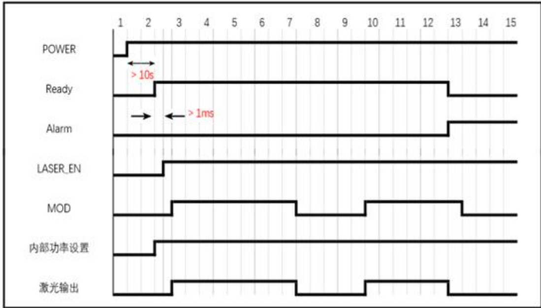
图 17 外控 RS232 控制方式连续模式时序图
