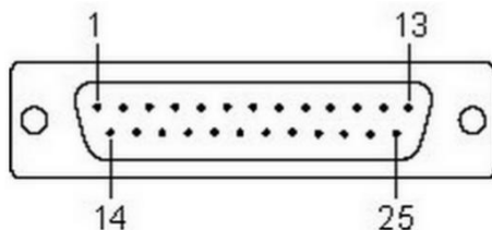
图 11 DB25 控制接口
