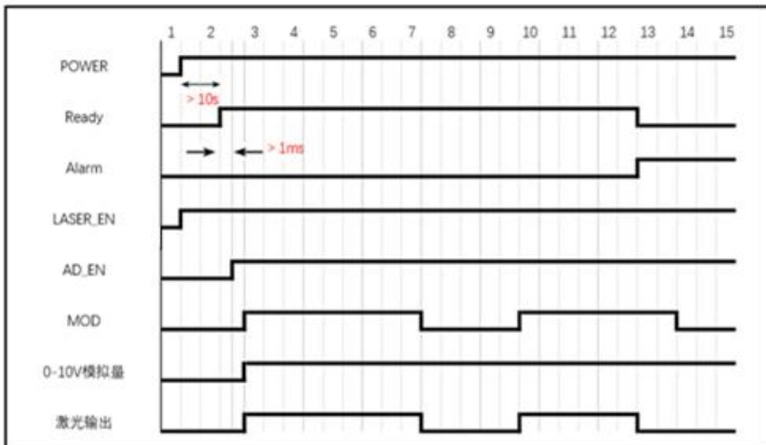
图 20 外控 AD 控制方式时序图
