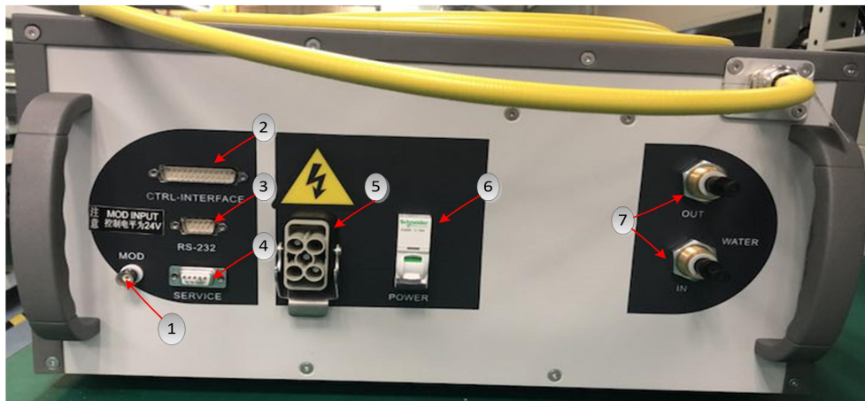
图 6 后面板
