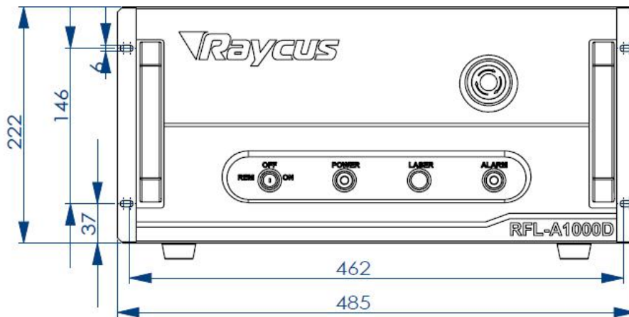
图2 激光器前视图 (单位: mm)
