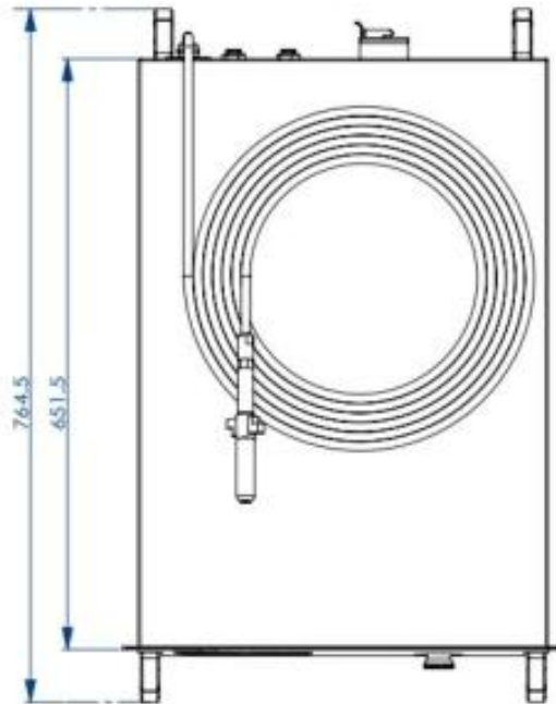
图 3b) 1500W/2000W 激光器俯视图(单位: mm)
