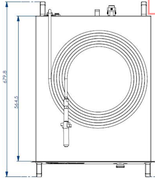
图 3a) 500W/1000W 激光器俯视图(单位: mm)
