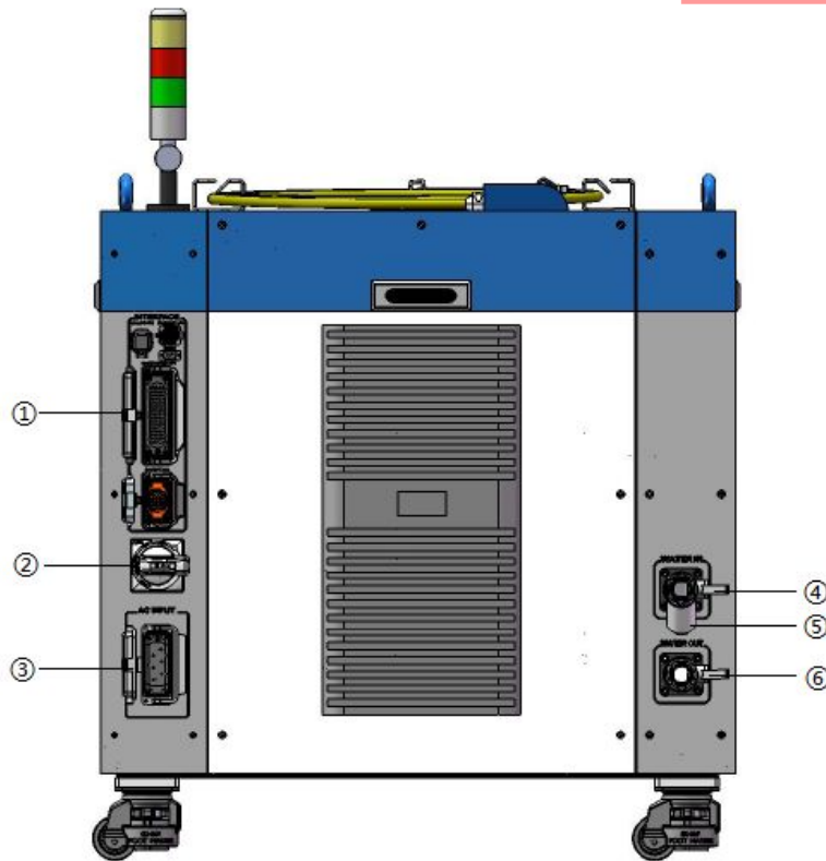
图 7 激光器后面板图
