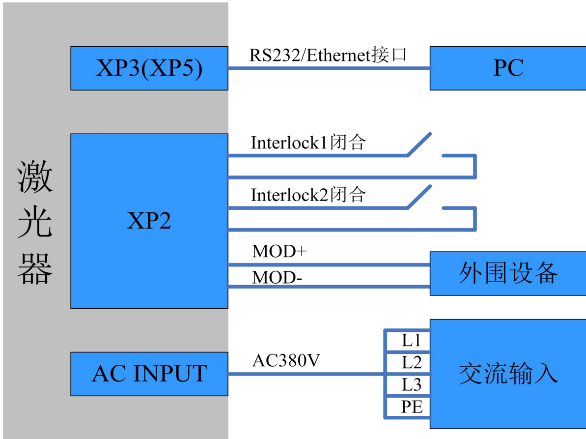
图 21 ON 模式下的功率通讯设置出光外控模式接线图
