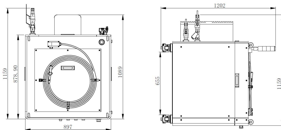
b)激光器俯视图及左视图
