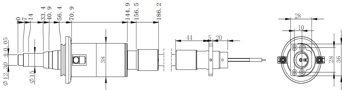
图 4 RFL-QD 输出光缆头外形尺寸图
