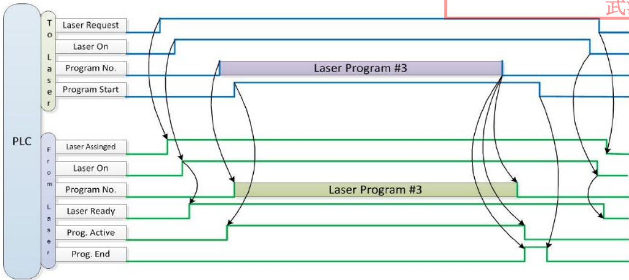
图 28 波形模式控制信号时序图
