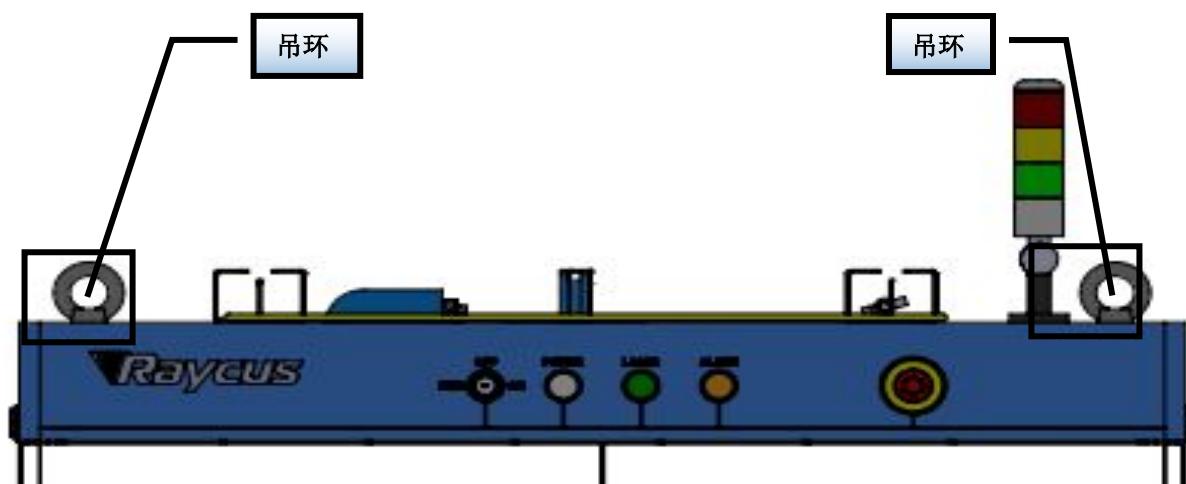
a) 吊环
