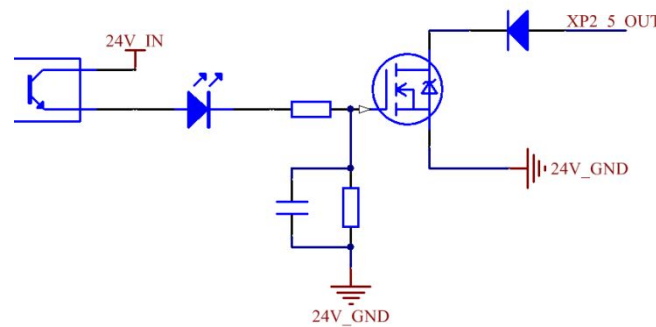
图 15 有源出光警告指示及主电源已上电警告指示电路图
