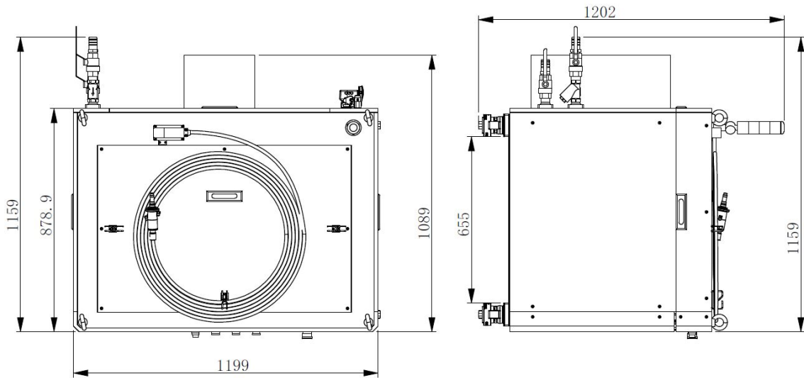
b)激光器俯视图及左视图
