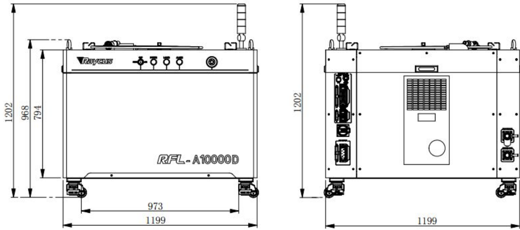
a)激光器前视图及后视图
