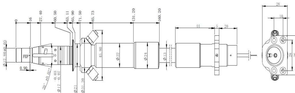
图 2 RFL- iHQB 输出光缆头外形尺寸图
