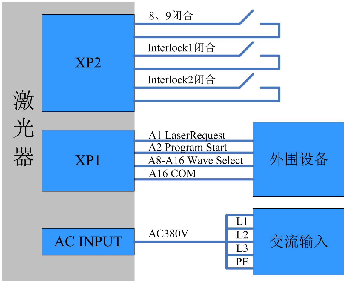
图 27 REM 模式下的波形模式接线图
