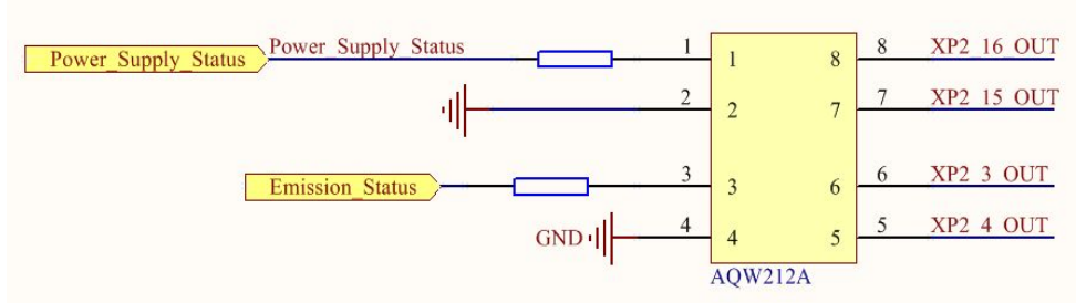
图 12 出光输出指示及主电源上电指示电路图
