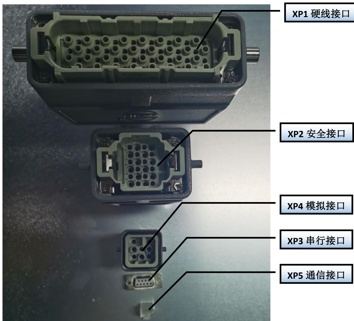
图 10 控制信号线
