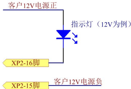
图 14 主电源已上电指示推荐的接线图（以 12V 为例）
