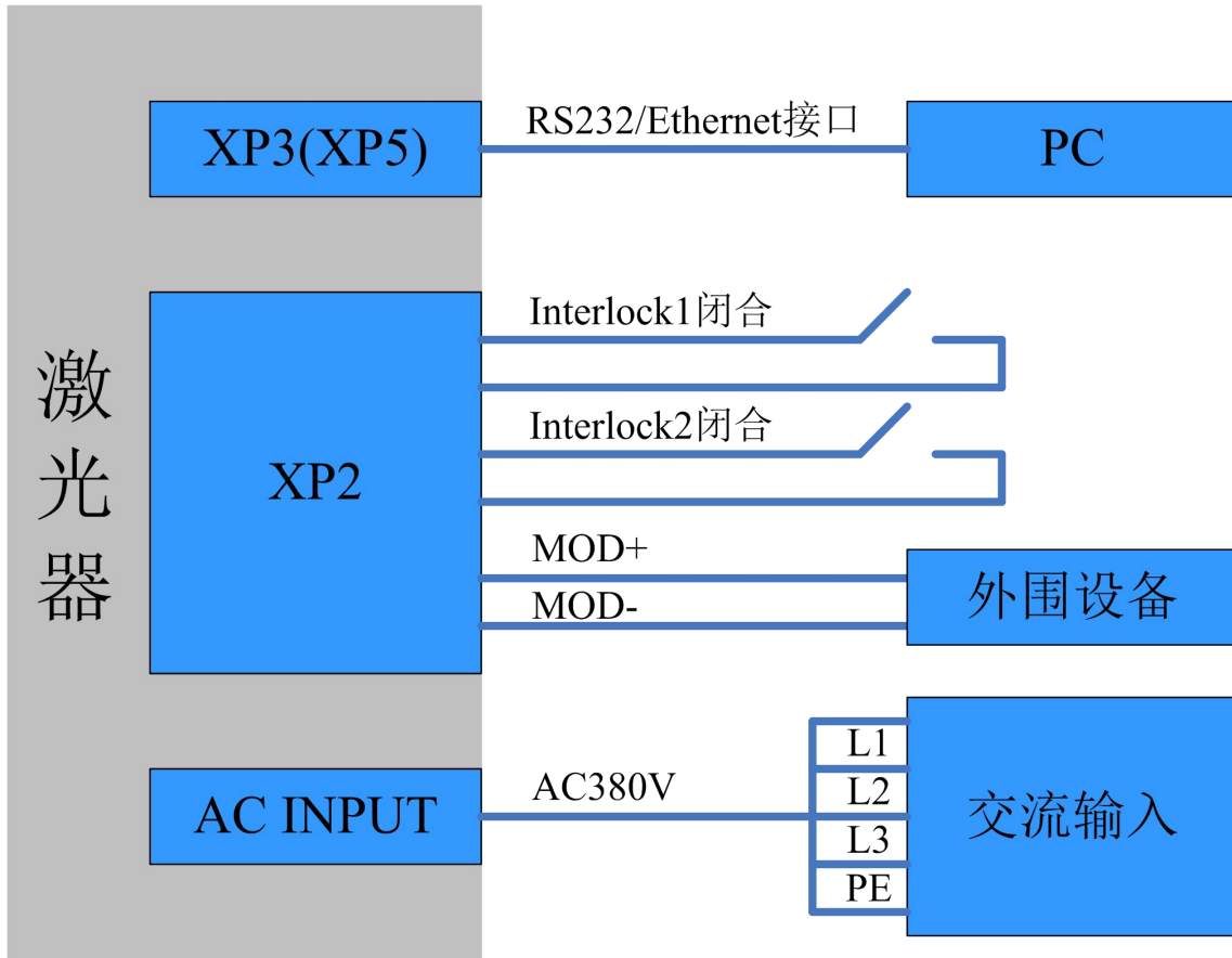
图 23 ON 模式下的波形模式外控出光接线图
