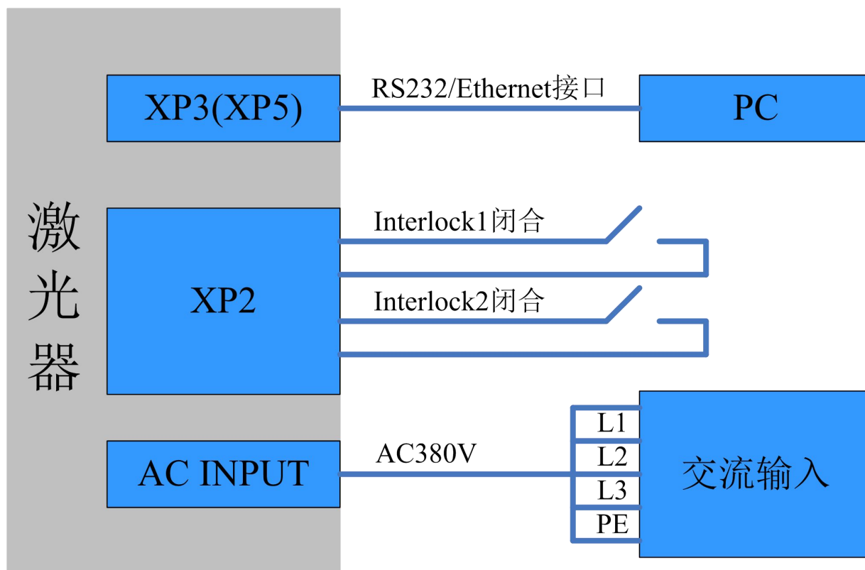
图 20 在“ON”模式下的接线图
