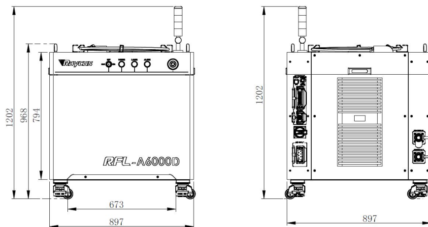
a)激光器前视图及后视图
