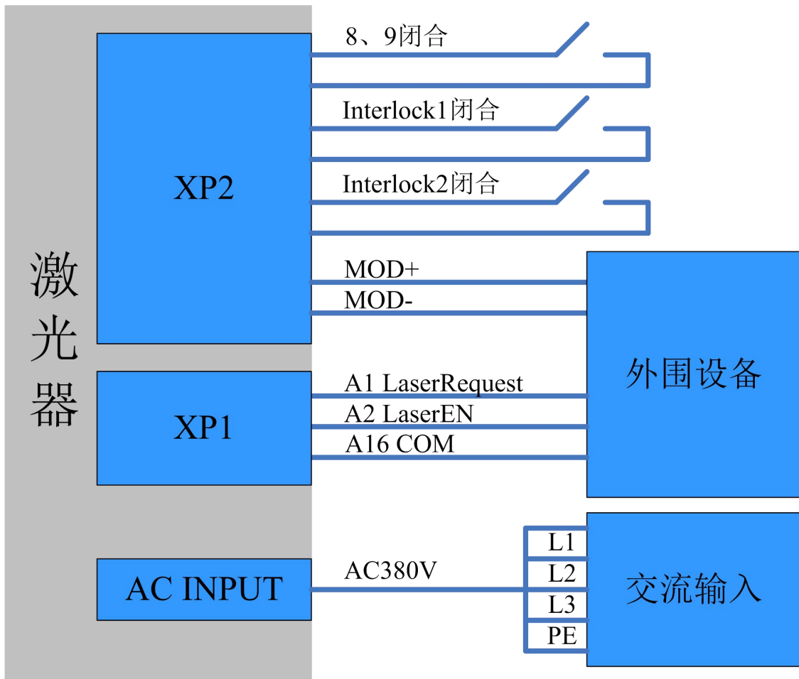
图 26 REM 模式下功率通讯设置出光外控接线图
