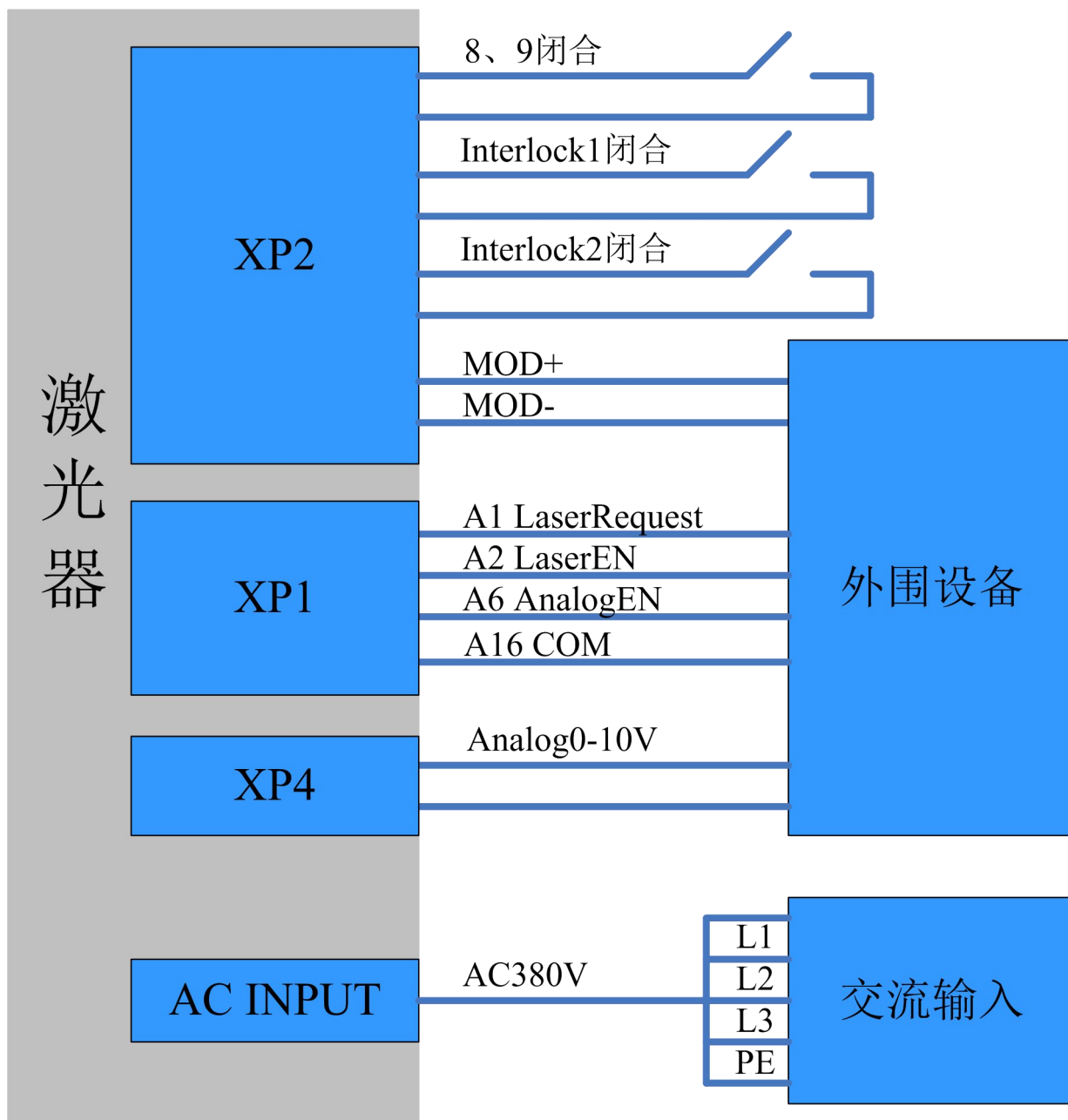
图 24 REM 模式下功率模拟量设置出光外控接线图
