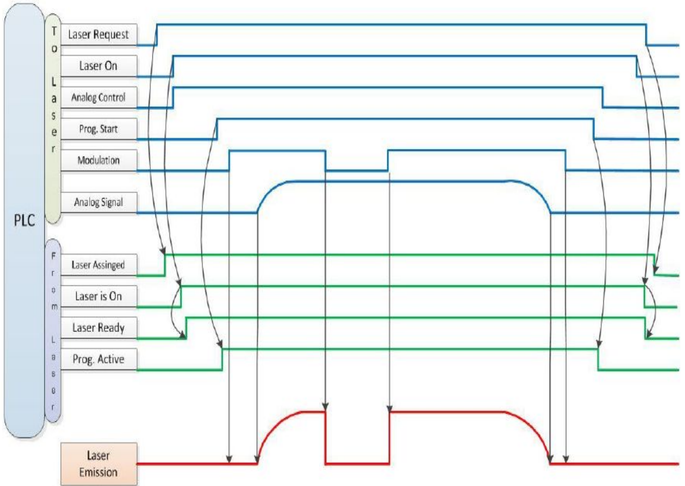
图 25 REM 模式下功率模拟量设置出光外控信号时序图
