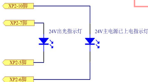
图 16 有源出光指示及主电源已上电指示推荐接线图
