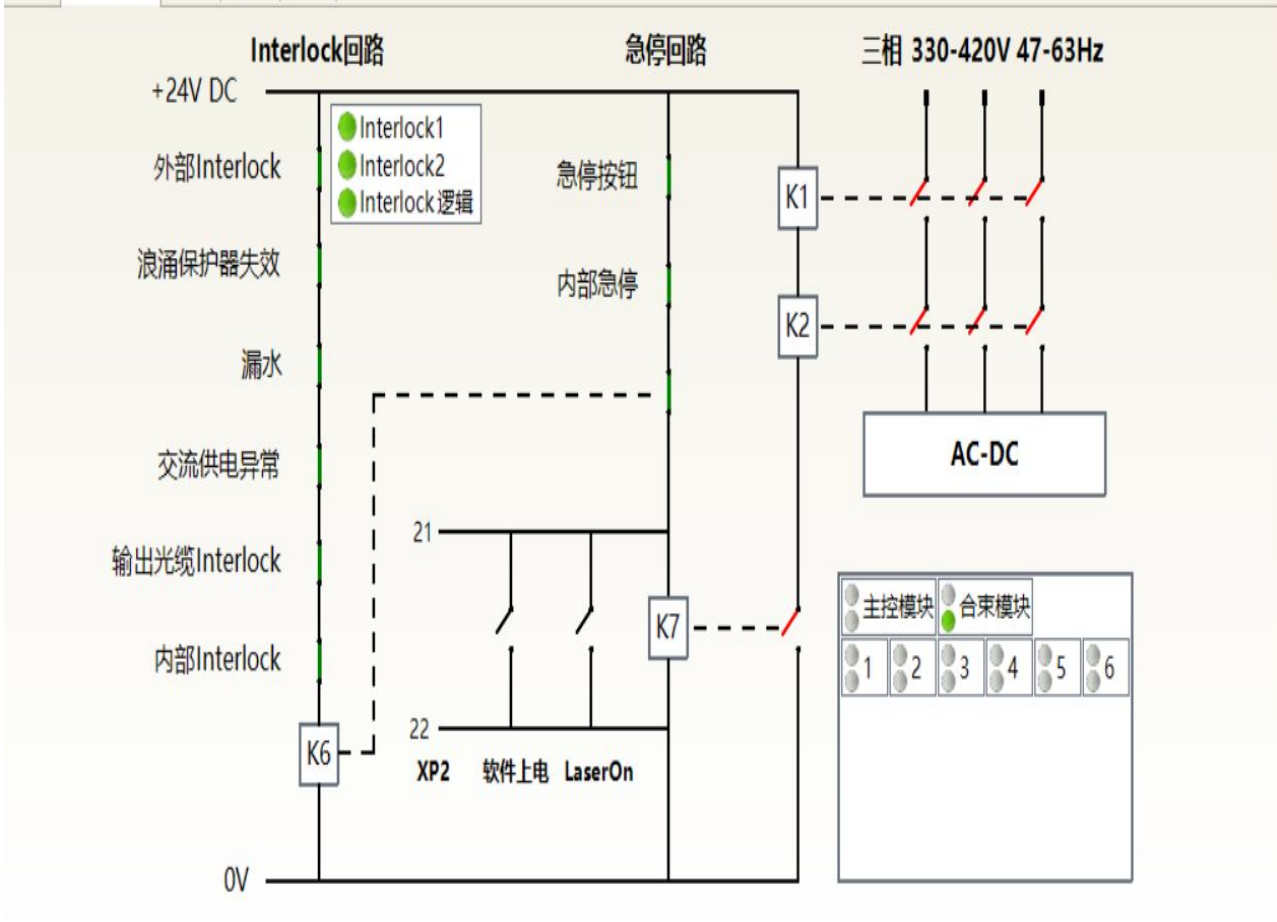
图 19 激光器内部电气回路示意图
