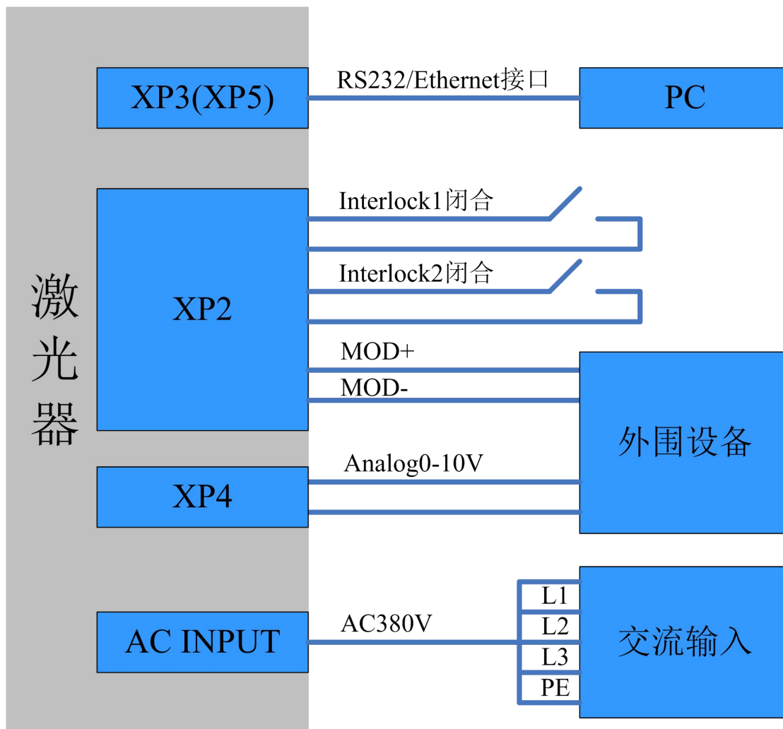
图 22 ON 模式下功率模拟量设置出光外控接线图
