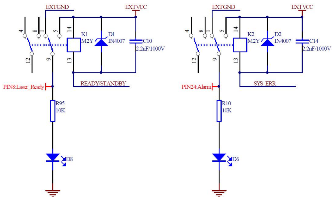
图 13 PIN 8、24 内部电路图
