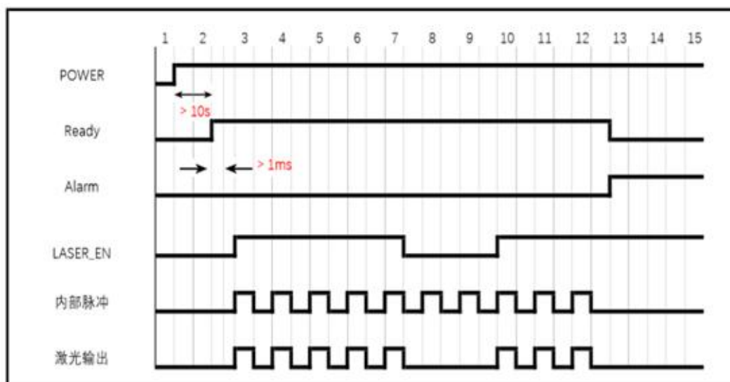
图 24 内控控制方式调制模式时序图
