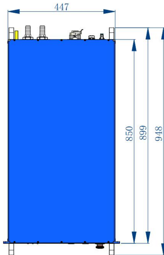
图 3 激光器俯视图(单位: mm)
