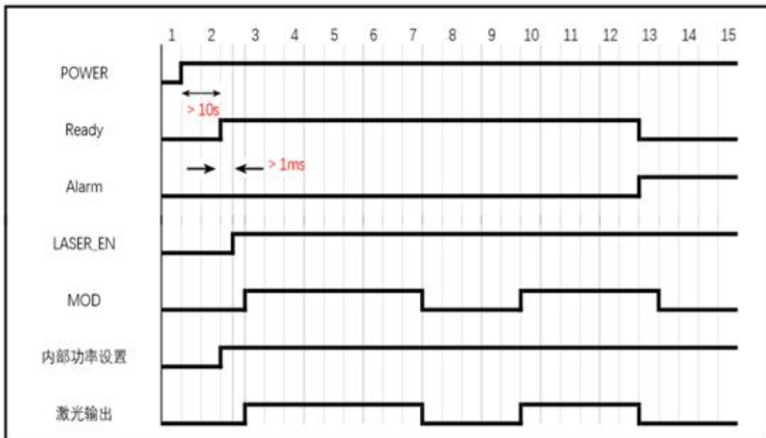
图 18 外控 RS232 控制方式连续模式时序图
