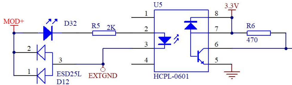
图 10 调制信号内部电路
