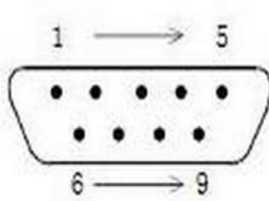
图 14 RS-232 串口示意图
