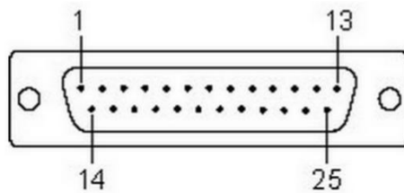
图 11 DB25 控制接口
