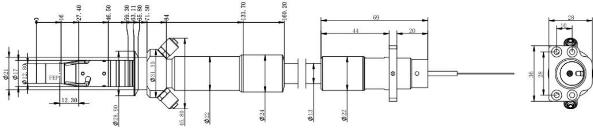
图 4 iHQB 输出头（单位：mm）
