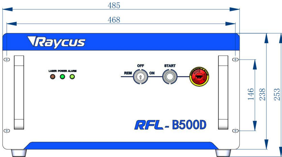
图 2 激光器外形尺寸及安装尺寸图。
