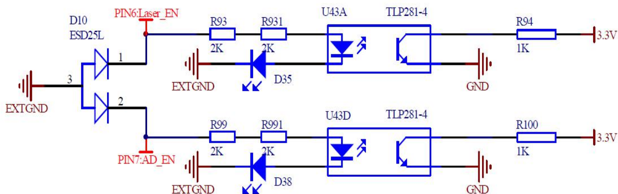
图 12 PIN 6、7 内部电路图
