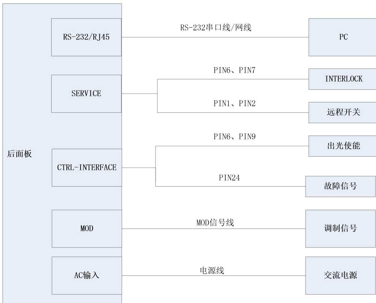
图 17 激光器外控 RS232 控制方式接线图
