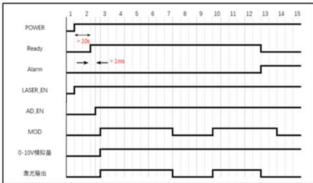
图 21 外控 AD 控制方式时序图
