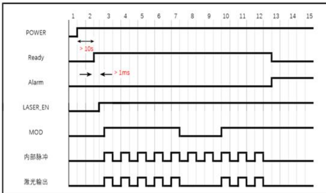
图 19 外控 RS232 控制方式调制模式时序图
