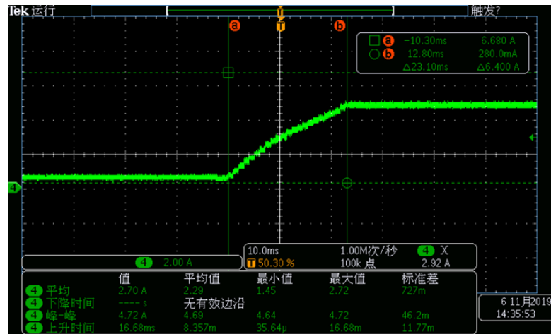
图 46 缓升波形
