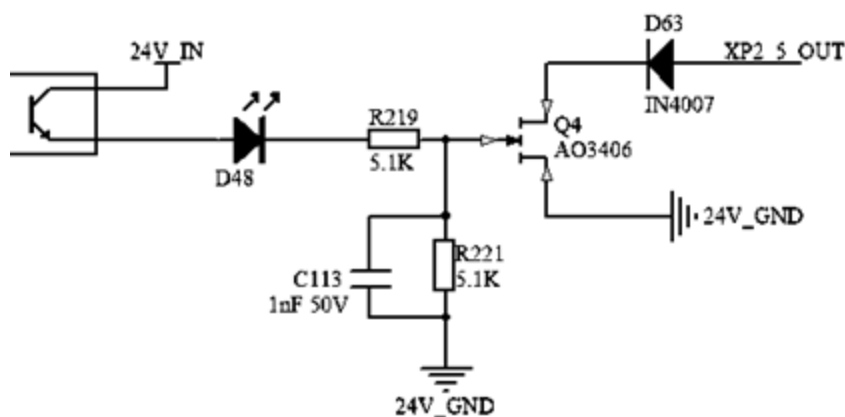
图 16 内部电路图
