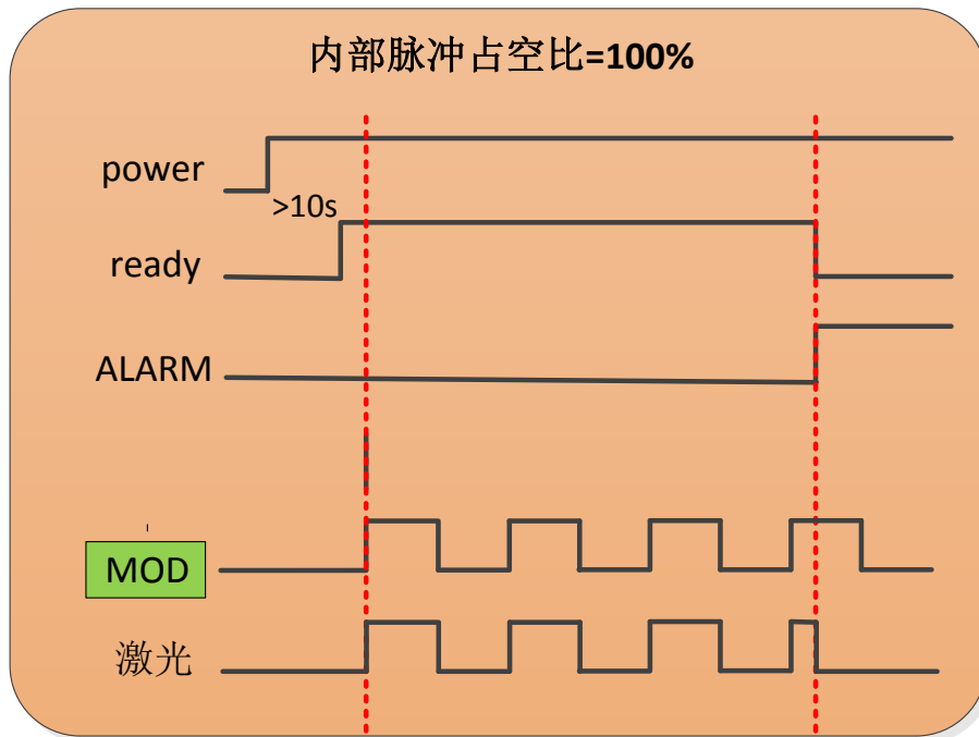
图 49 内部脉冲占空比为 100%时激光器的输出波形
