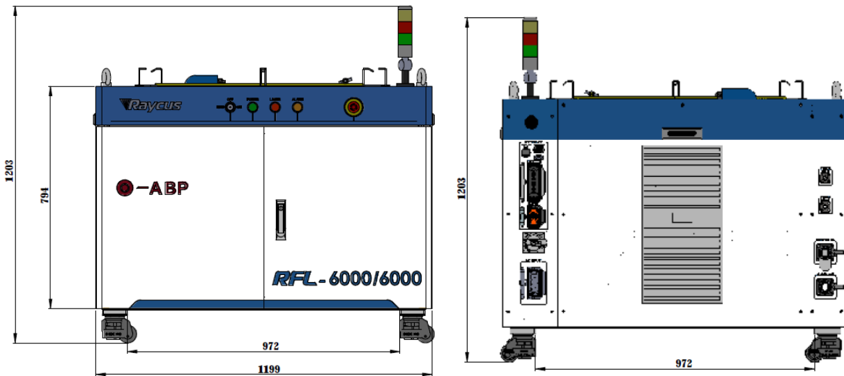
a) 激光器前视图及后视图
