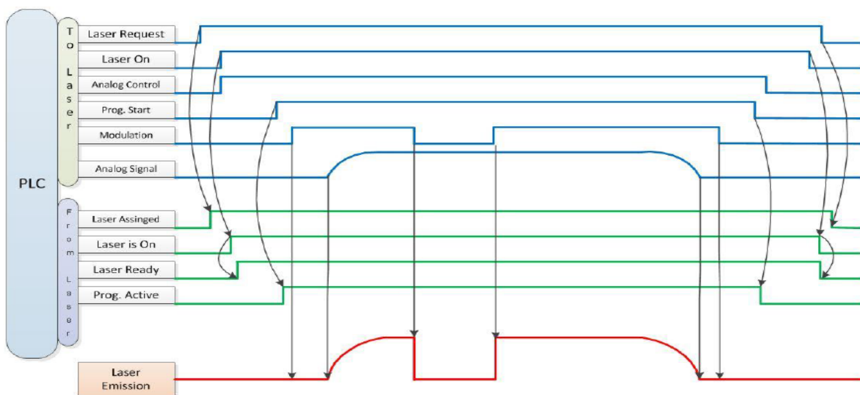
图 26 时序图
