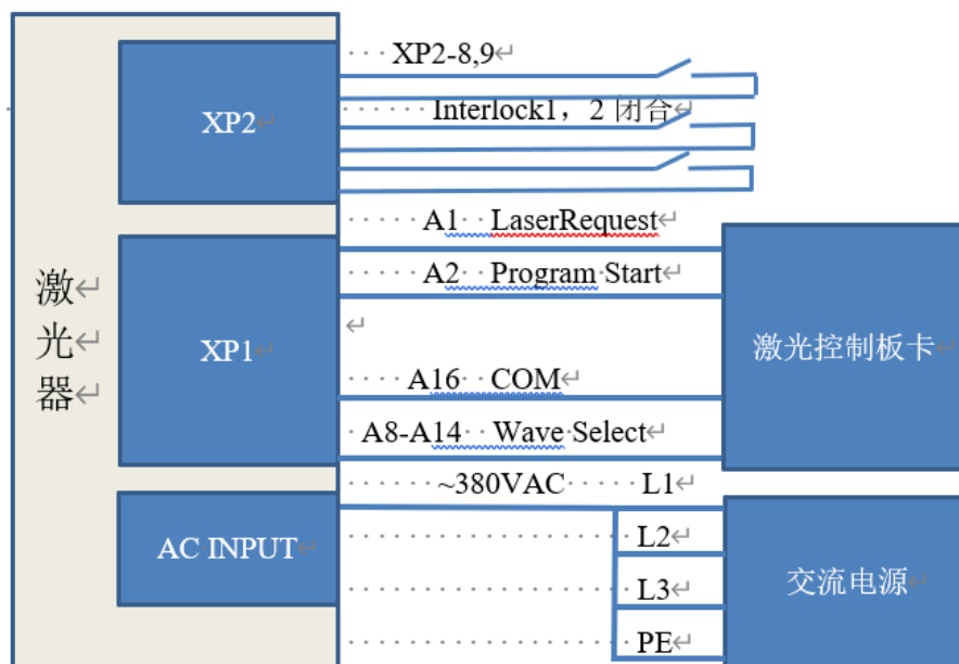
图 28 REM 模式下编程模式接线图
