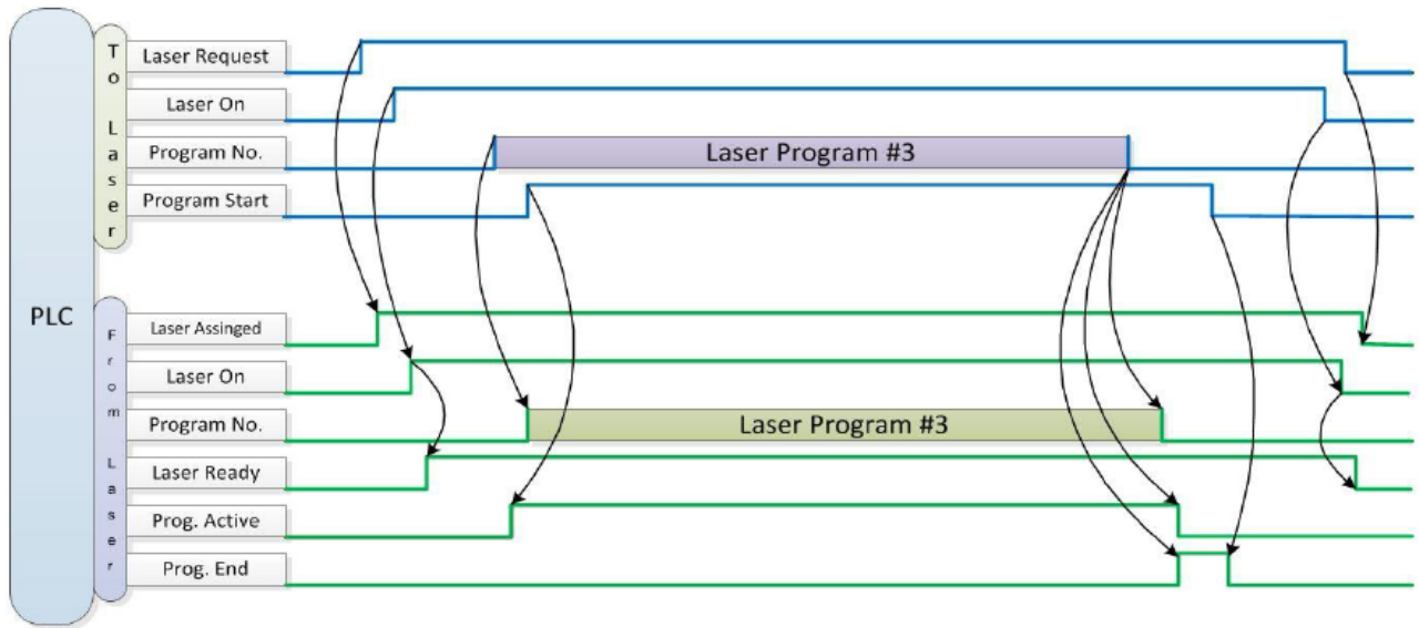
图 29 时序图
