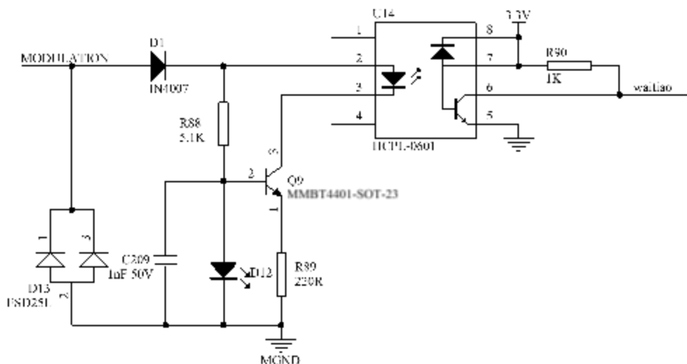
图 13 MOD 信号原理图
