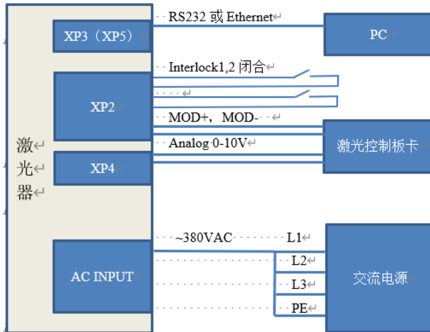
图 23 ON 模式下功率出光皆外控接线图
