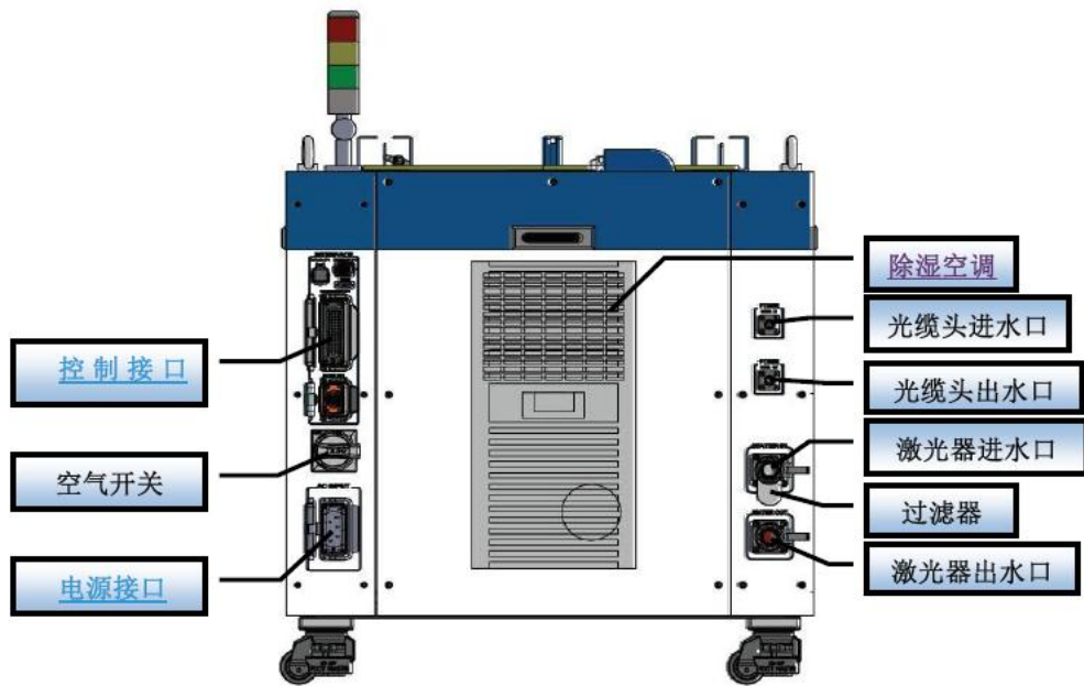
b) 3000/3000, 4000/2000, 2000/4000, 4000/4000 激光器后面板
