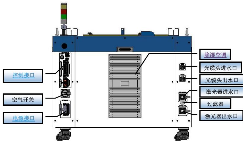
c) 6000/6000 激光器后面板
