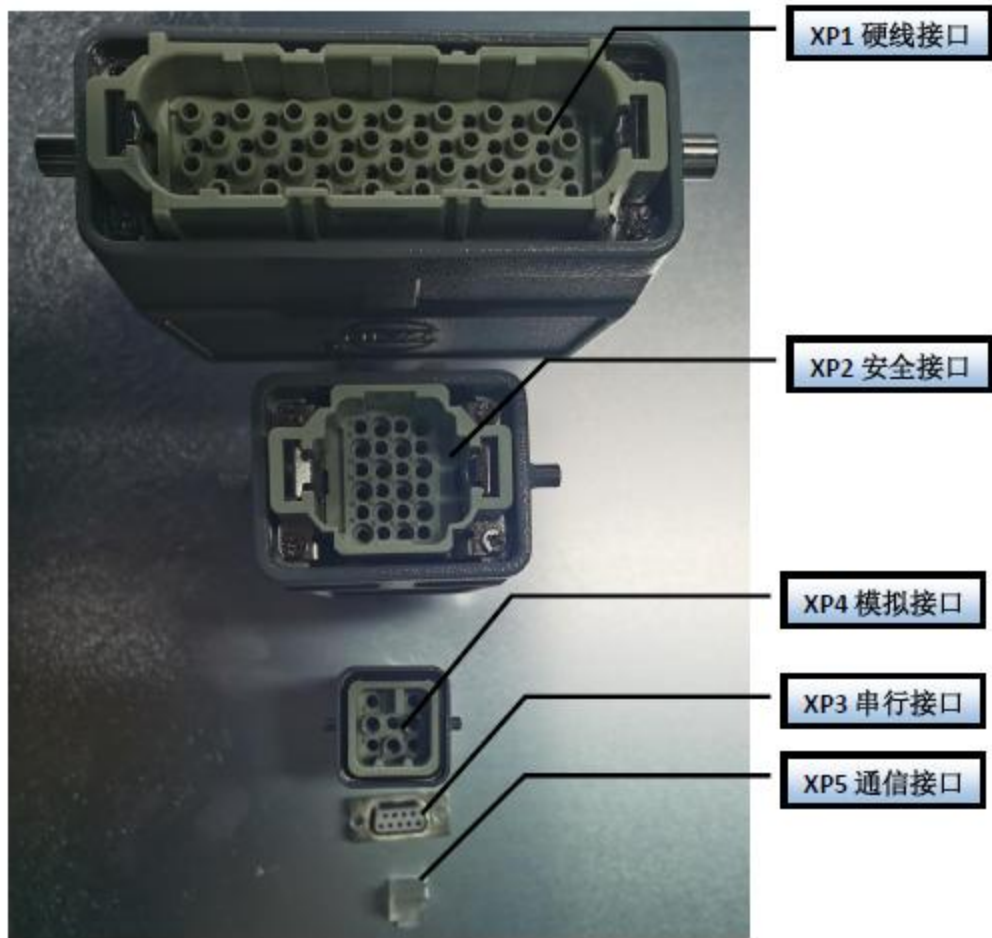
图 12 控制信号线
