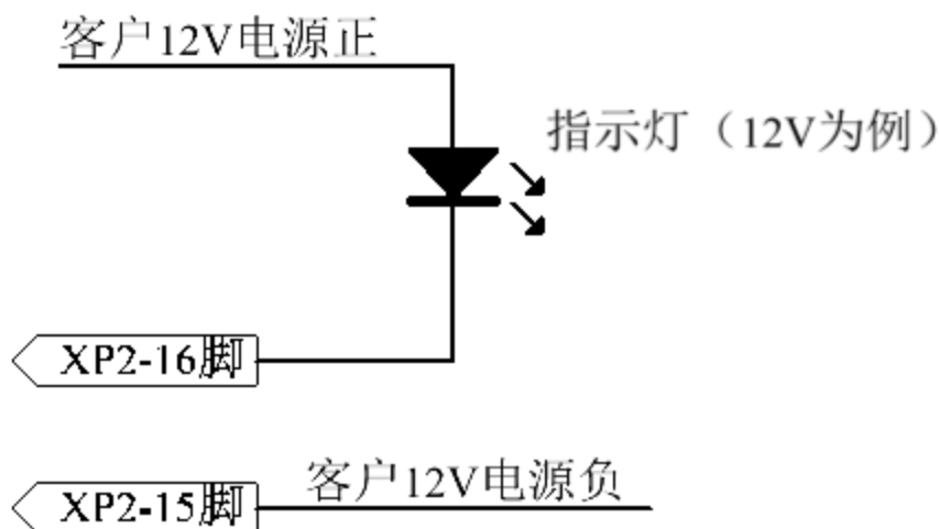
图 15 推荐接线方法
