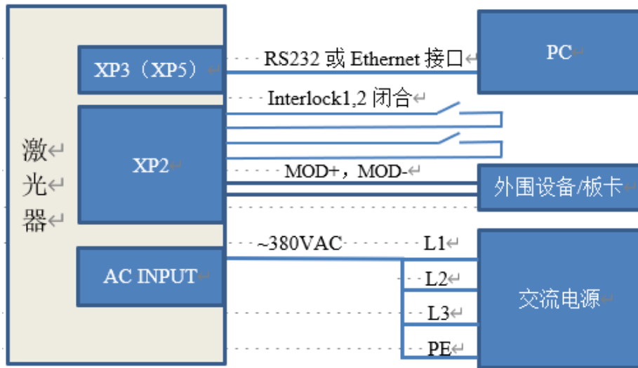
图 22 ON 模式下功率内控、外控出光接线图
