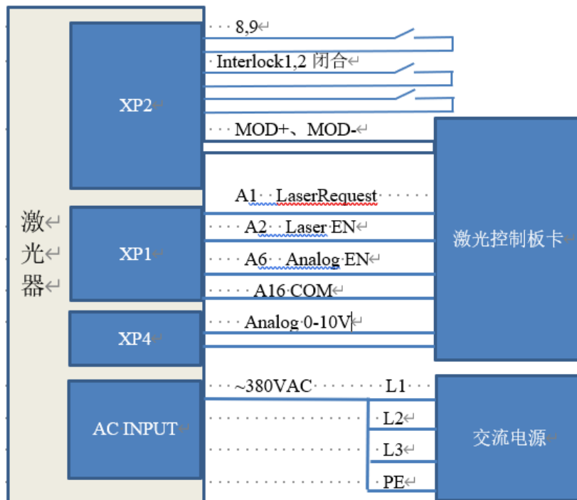
图 25 REM 模式功率出光皆外控接线图
