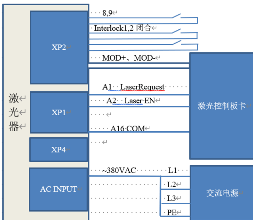
图 27 REM 模式下功率内控、出光外控接线图
