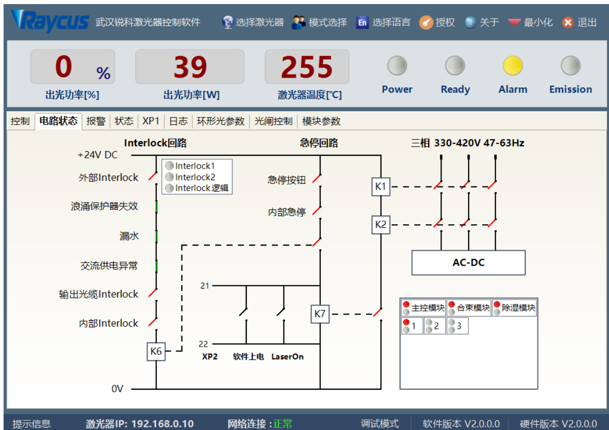
图 20 激光器内部电气回路示意图
