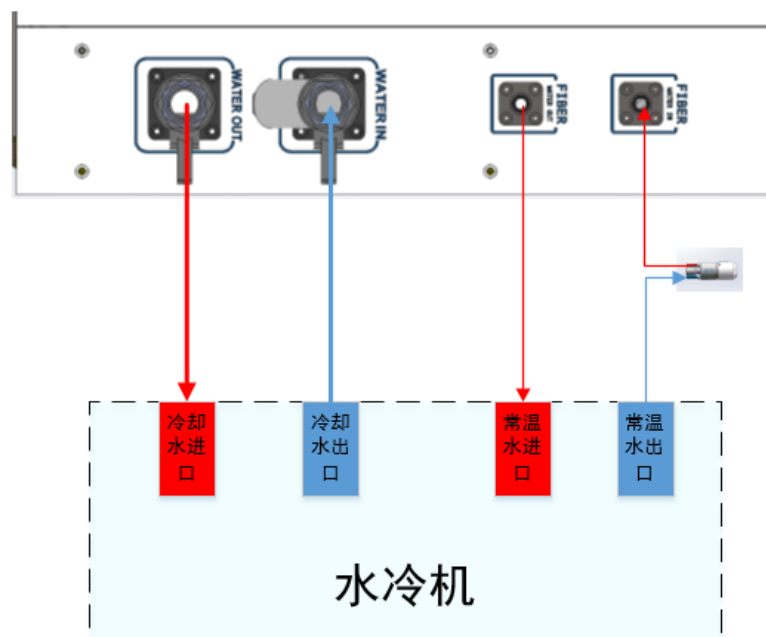
图 7 激光器冷却系统连接示意图
