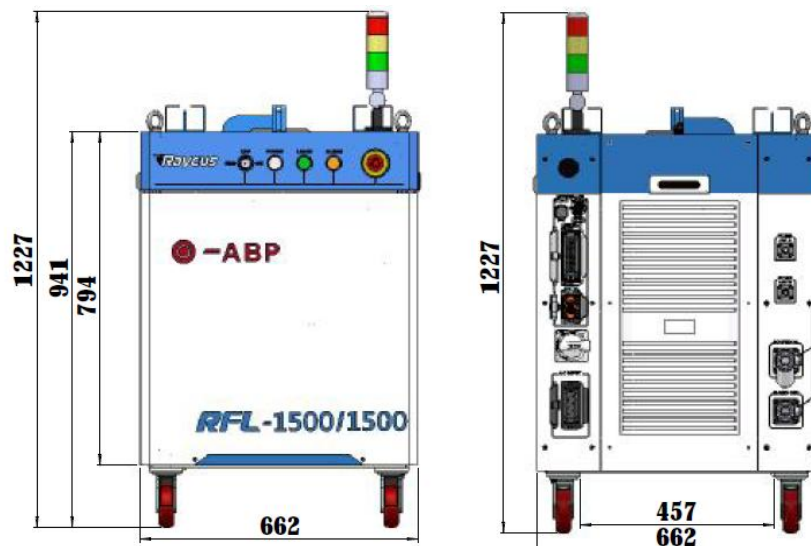
a) 激光器前视图及后视图
