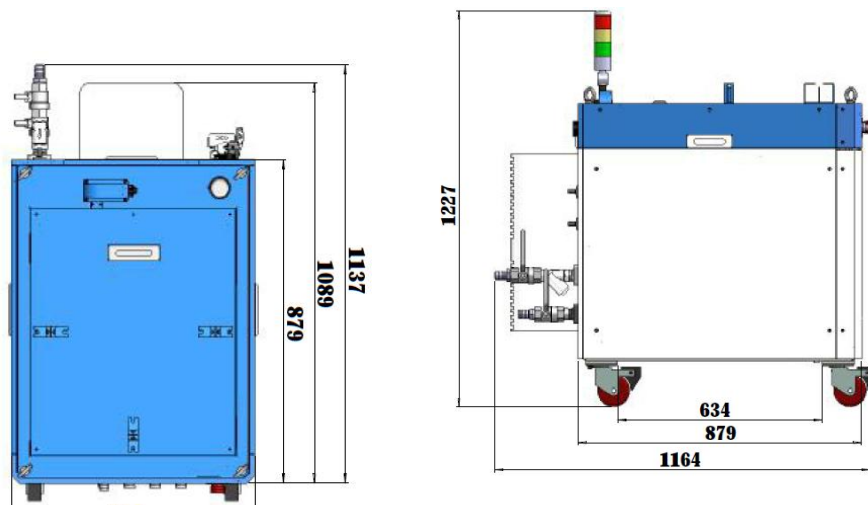
b) 激光器俯视图及左视图
