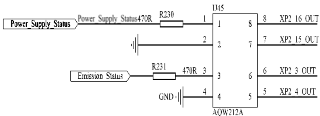
图 14 内部原理图
