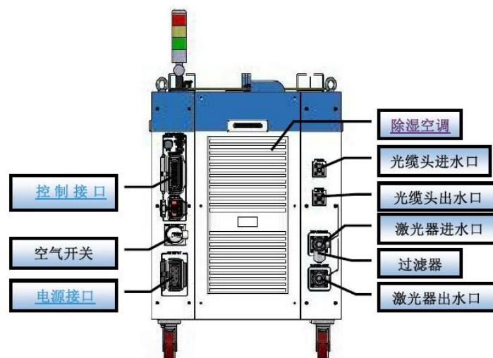
a) 1500/1500, 2000/2000 激光器后面板
