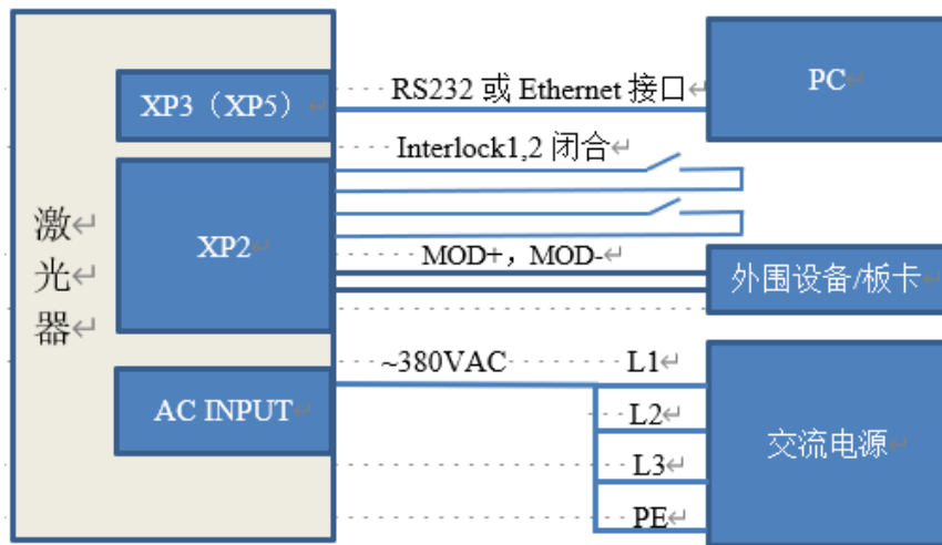
图 24 ON 模式下编程模式外控出光接线图
