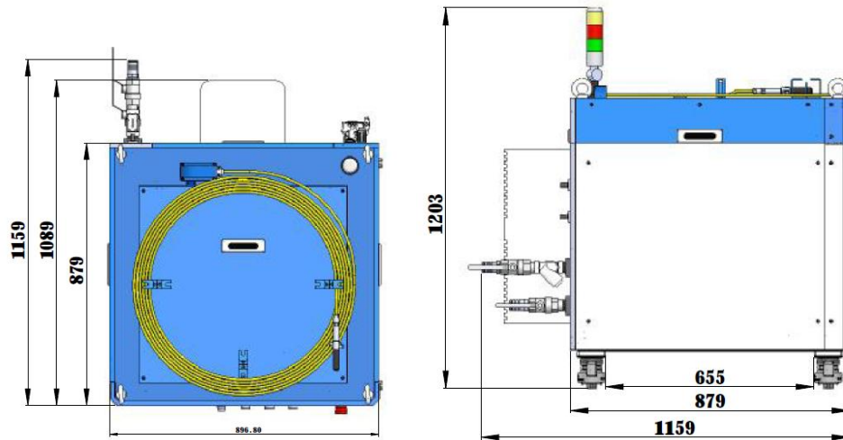
b) 激光器俯视图及左视图
