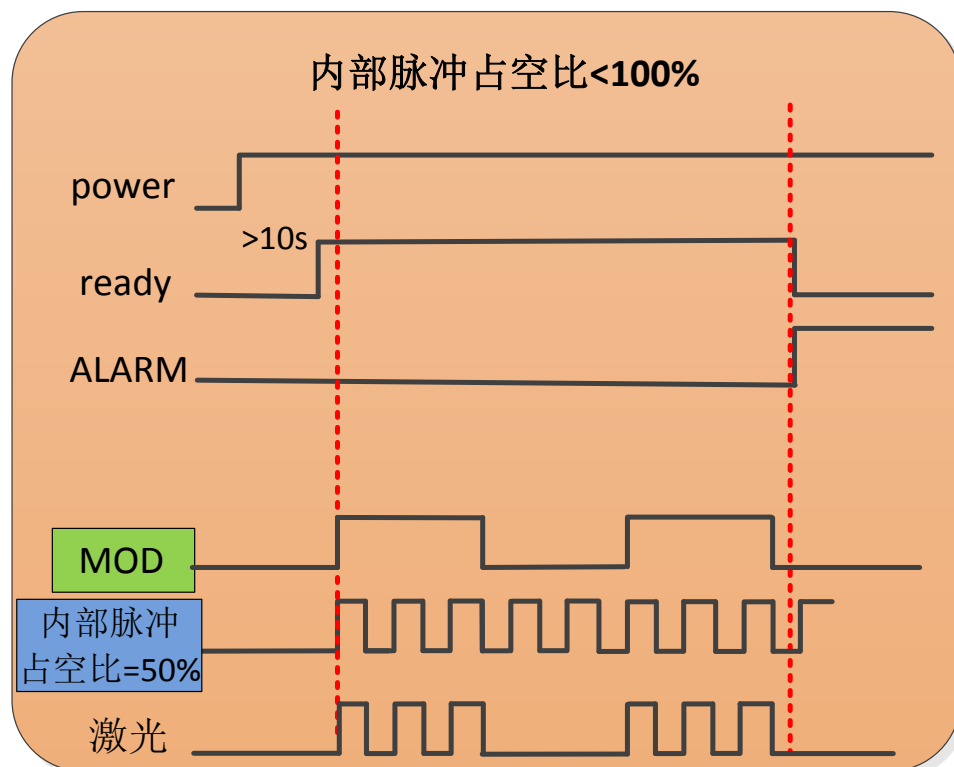
图 50 内部脉冲占空比小于 100%时激光器的输出波形
