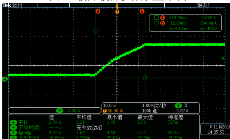
图 50 缓升波形
