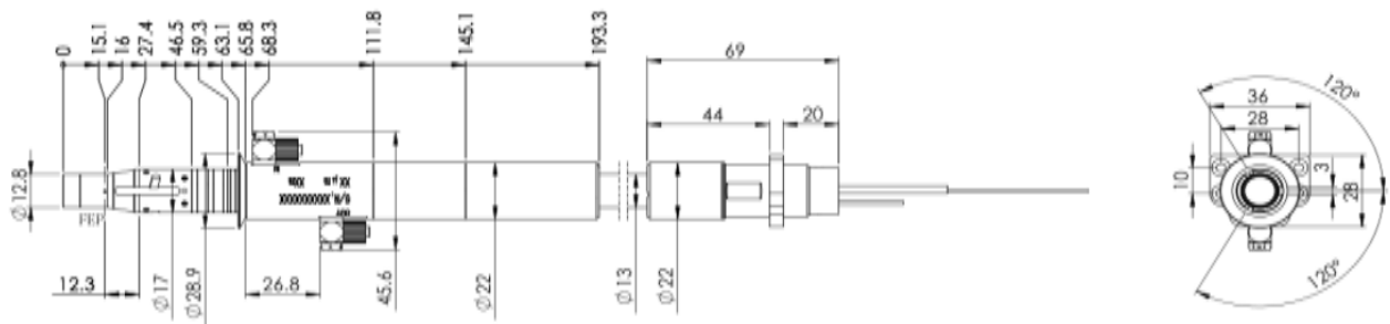
图 3（a） QBH 输出光缆头外形尺寸图
