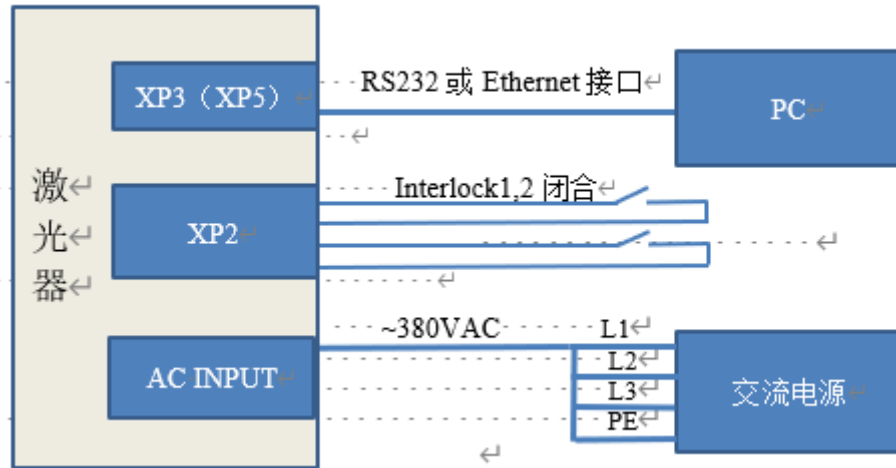
图 25 钥匙开关“ON”软件模式下内控接线图
