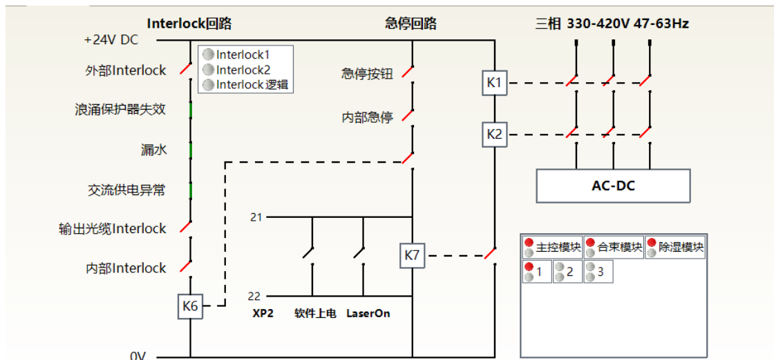
图 23 激光器内部电气回路示意图
