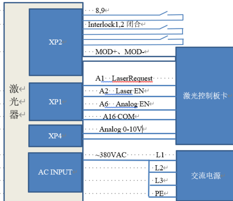
图 29 REM 模式功率出光皆外控接线图
