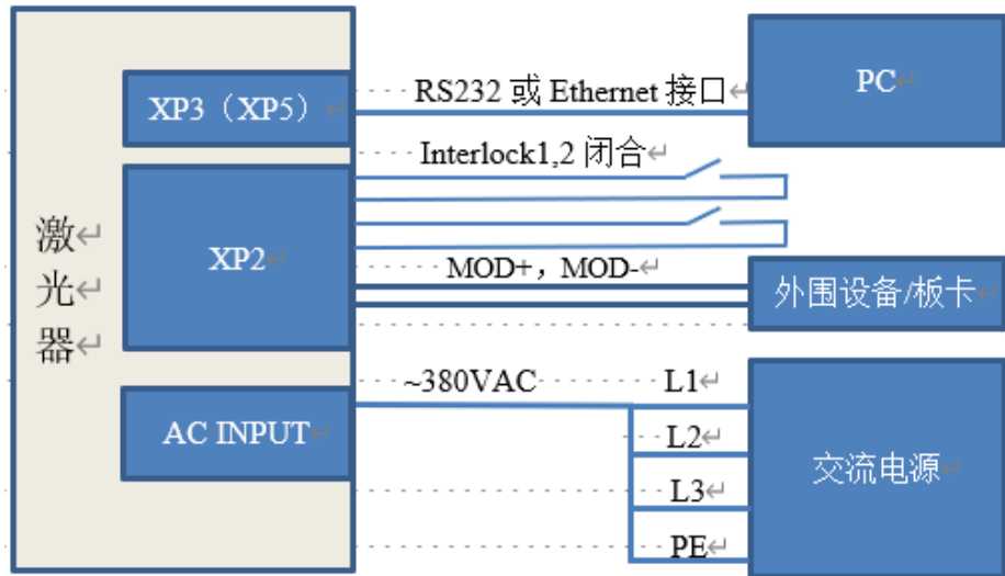
图 26 ON 模式下功率内控、外控出光接线图
