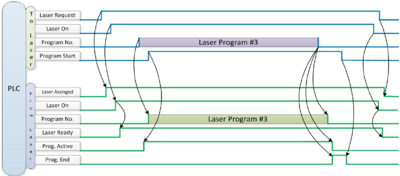
图 33 时序图
