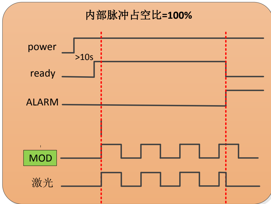
图 54 内部脉冲占空比为 100%时激光器的输出波形 当占空比小于 100%时，实际出光等于外部 MOD 信号跟内部的频率的相与。
