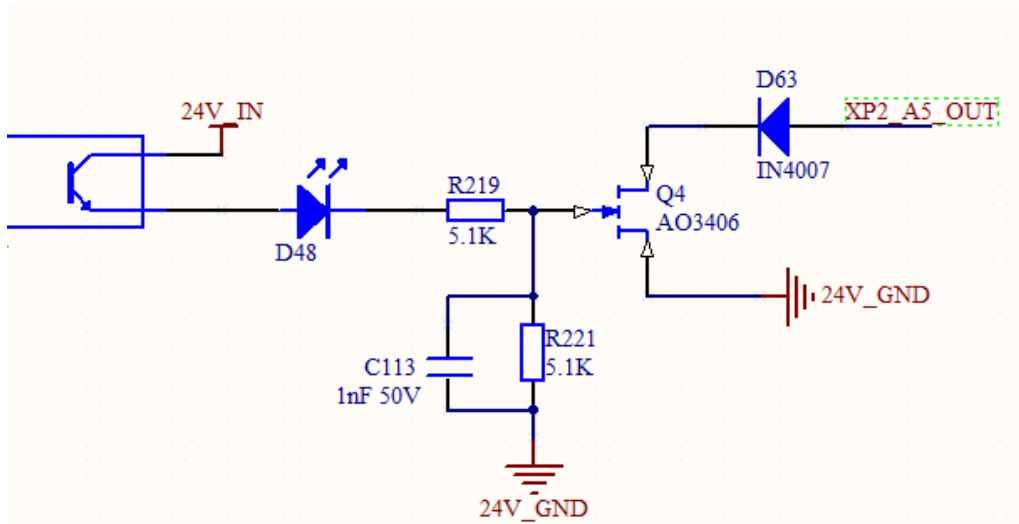
图 19 内部电路图
