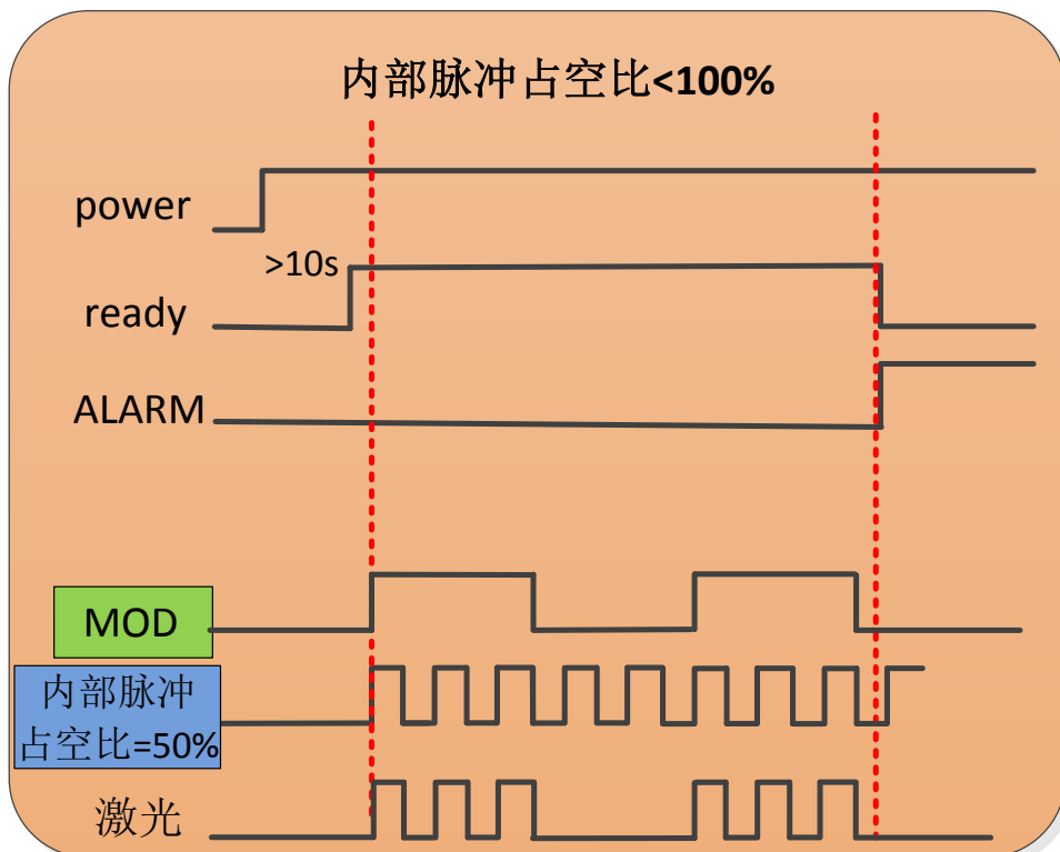
图 55 内部脉冲占空比小于 100%时激光器的输出波形
