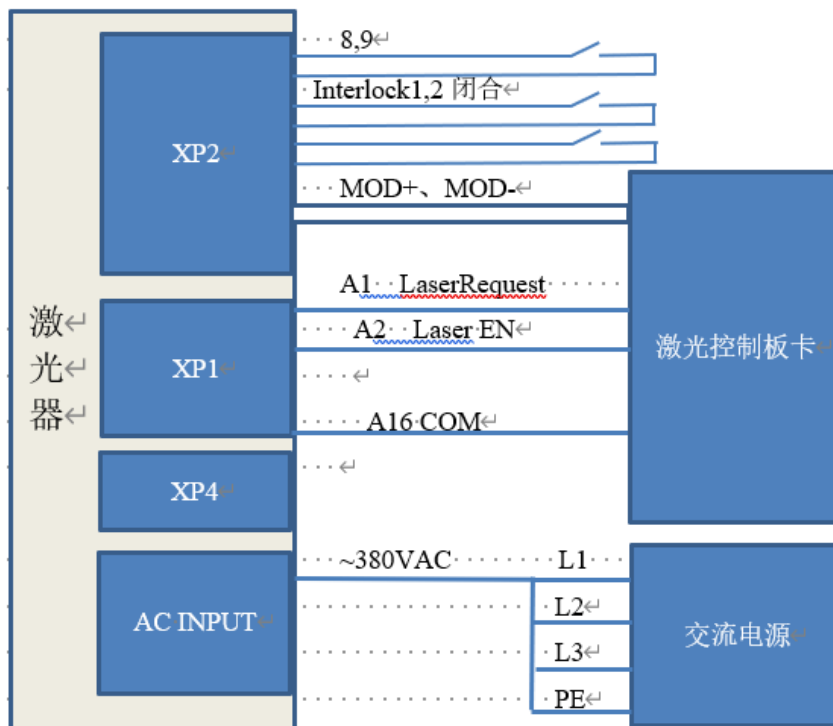
图 31 REM 模式下功率内控、出光外控接线图
