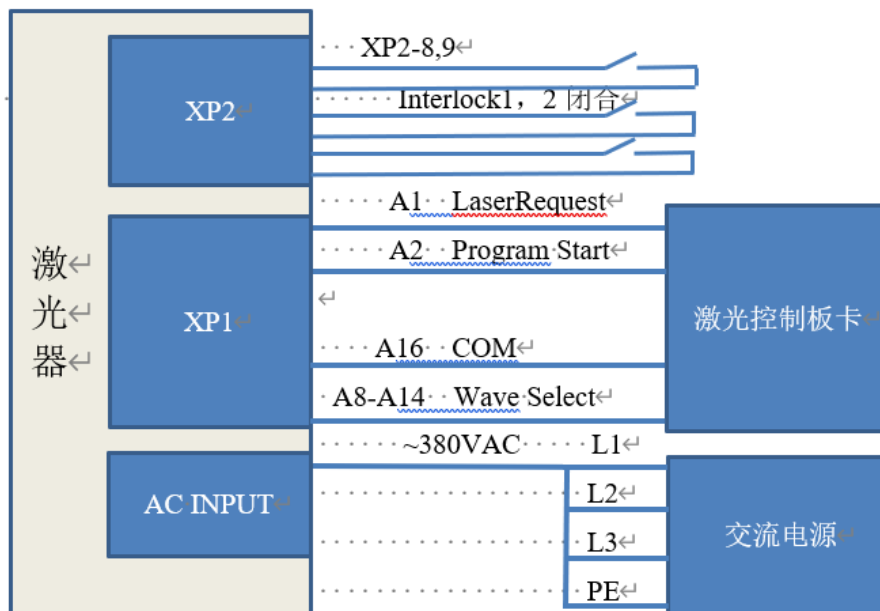
图 32 REM 模式下编程模式接线图
