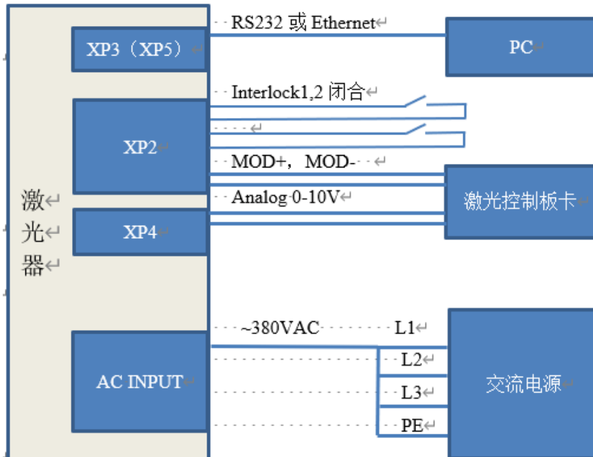
图 27 ON 模式下功率出光皆外控接线图
