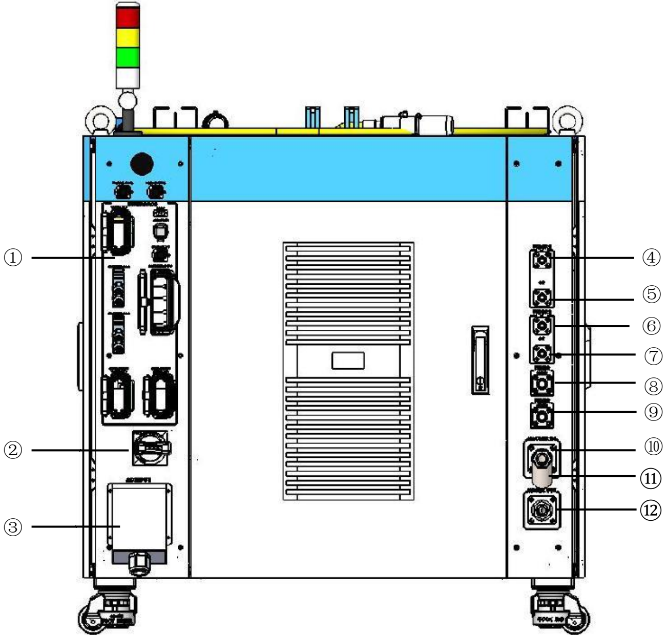
图 13 激光器后面板
