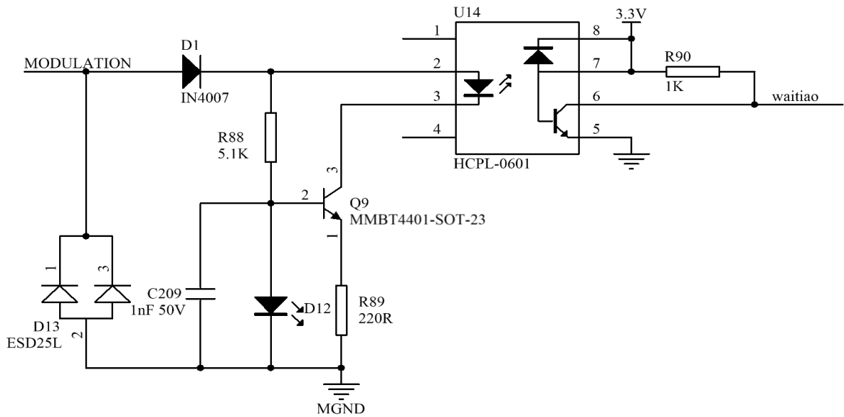
图 16 MOD 信号原理图
