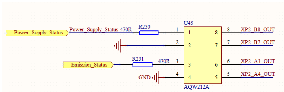
图 17 内部原理图
