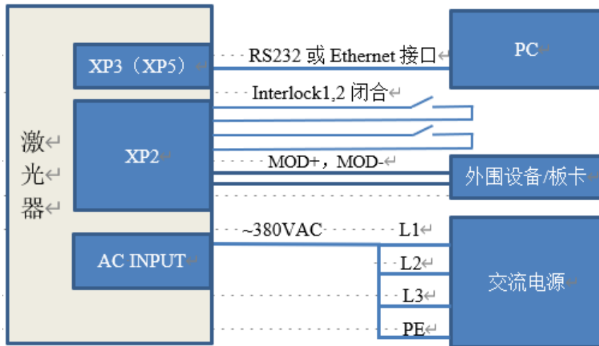
图 28 ON 模式下编程模式外控出光接线图
