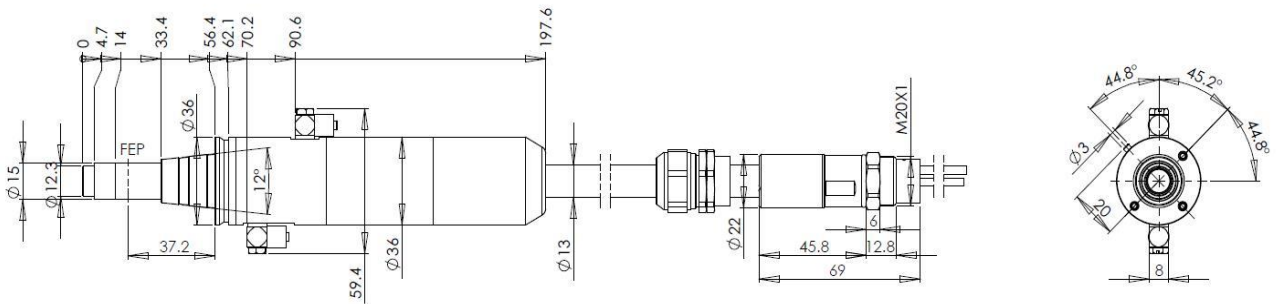
图 3 (b) QD 输出光缆头外形尺寸图
