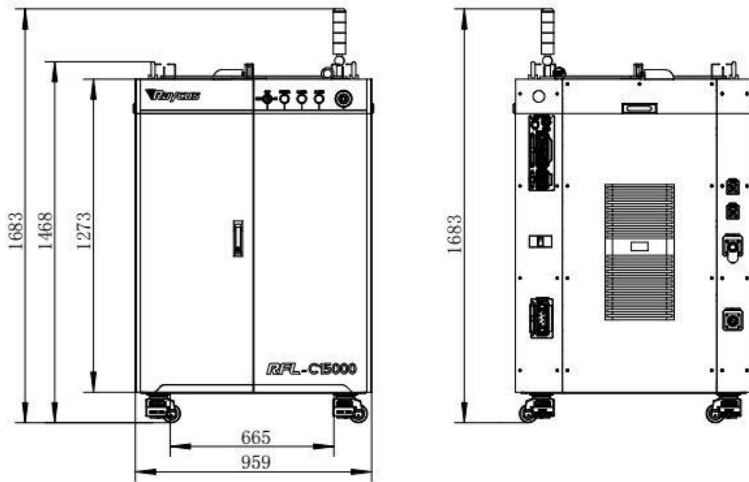
a)激光器前视图及后视图
