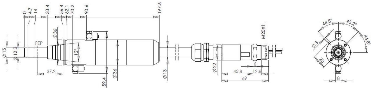
图 2 RFL-QD 输出光缆头外形尺寸图
