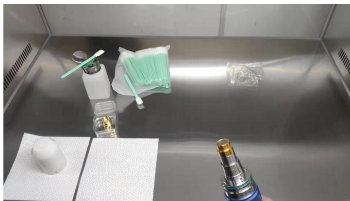
图 8 取下白色防尘盖的输出光缆
