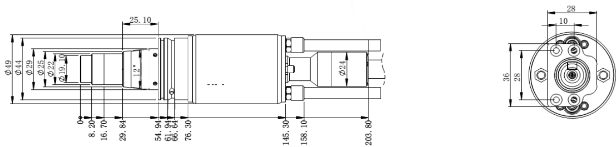
a) RFL-QP 输出光缆头外形尺寸图 (RFL-C40000/50000)
