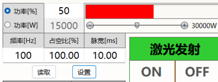
图 36 出光参数设置区显示界面
