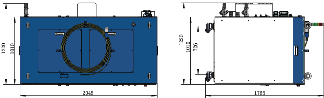
b) 激光器俯视图及左视图
