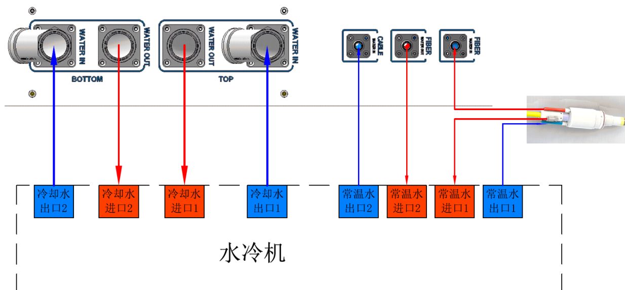
b) RFL-C60000 冷却水连接方式
