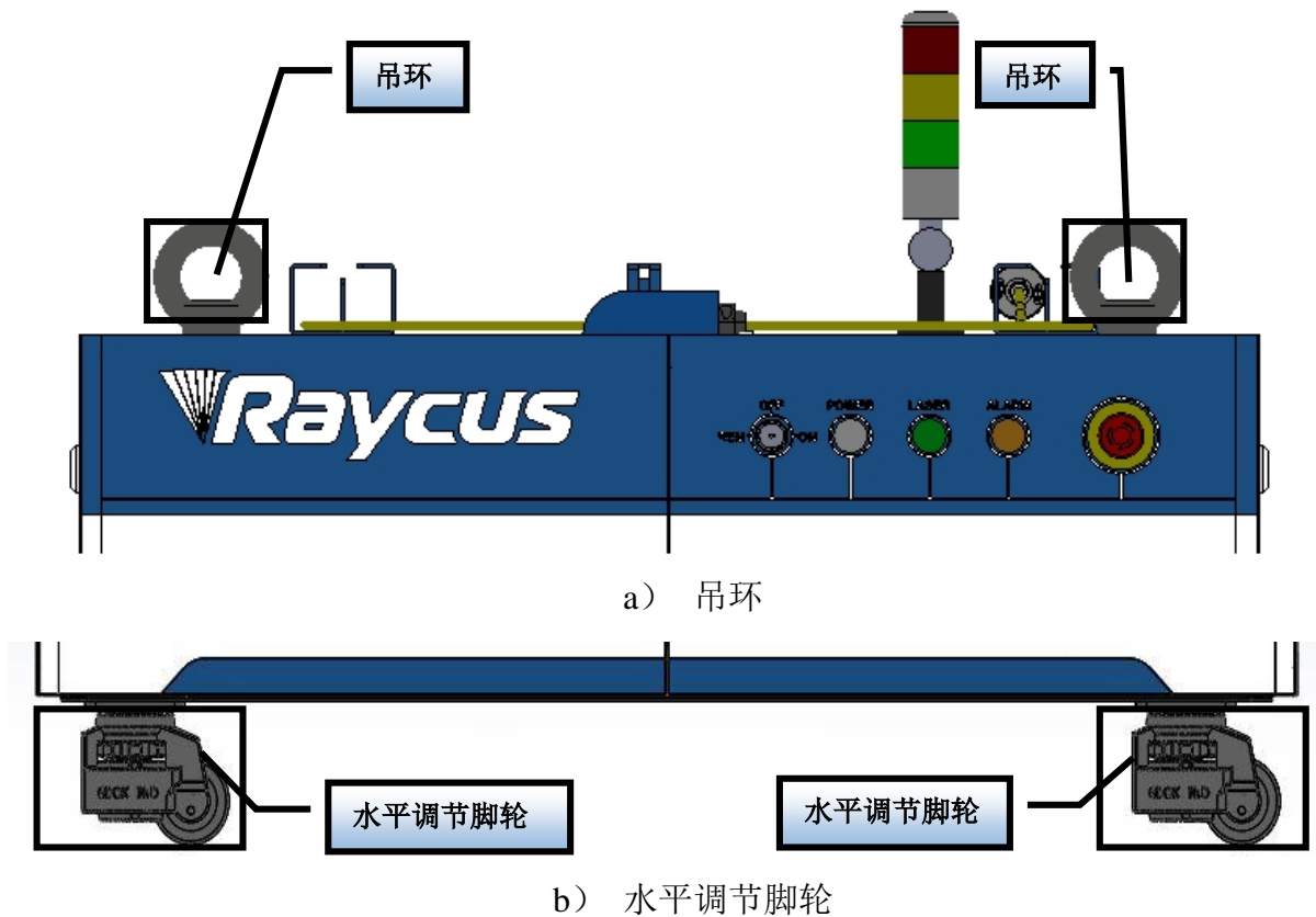
图 4 激光器顶部吊环及底部水平调节脚轮
