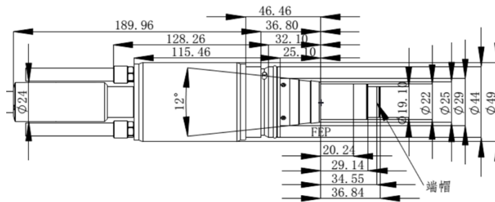
b) RFL-HQP 输出光缆头外形尺寸 (RFL-C60000)
