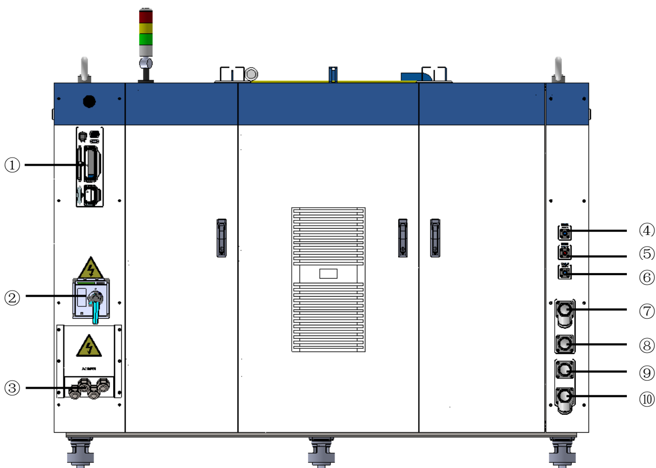
图 12 激光器后面板图
