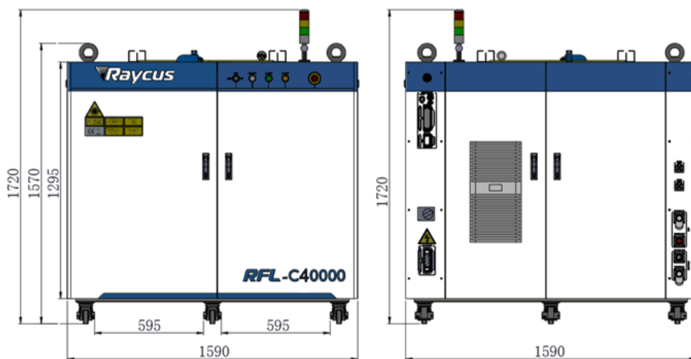
a) 激光器前视图及后视图
