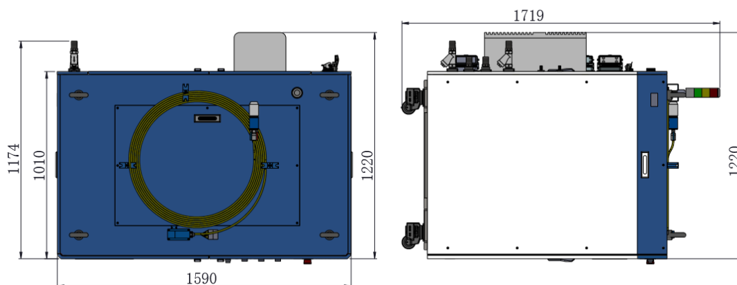
b) 激光器俯视图及左视图
