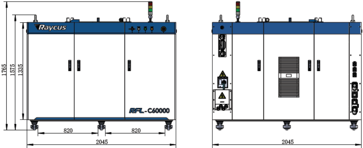
a) 激光器前视图及后视图
