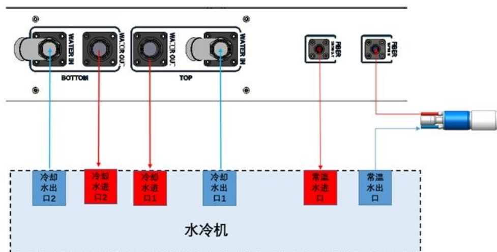
a) RFL-C40000/C50000 冷却水连接方式
