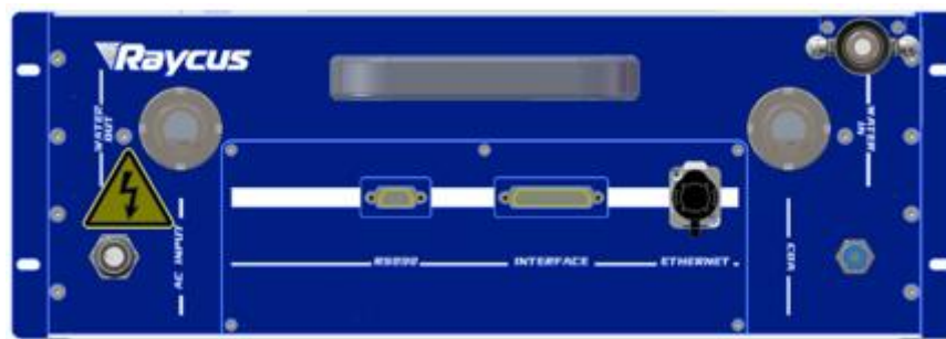
图 7 RFL-C6000S 激光器后面板
